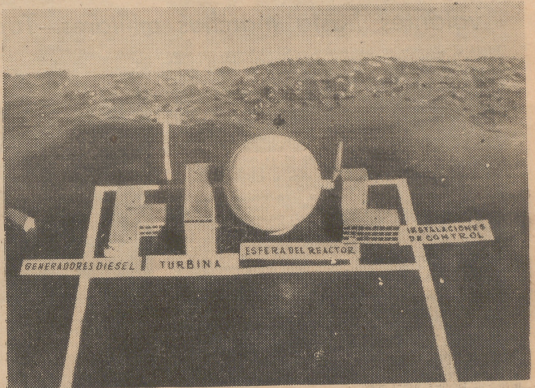
Esta es la maqueta de una nueva central de energía atómica, que será construida en Caithness (Escocia). Comprenderá un reactor capaz de desarrollar una gran energía calorífica y que convertirá el uranio ordinario en plutonio. La gran esfera central contendrá las sustancias radiactivas. Estas instalaciones suministrarán dentro de unos cinco años energía atómica para usos domésticos e industriales.
