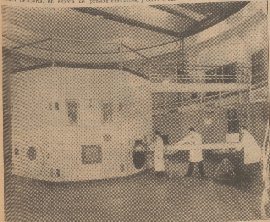
En el Laboratorio Nacional de Chicago ha sido instalado recientemente un nuevo reactor para investigaciones atómicas, que utiliza como "combustible" el uranio 235. Tiene cuatro metros y medio de altura
