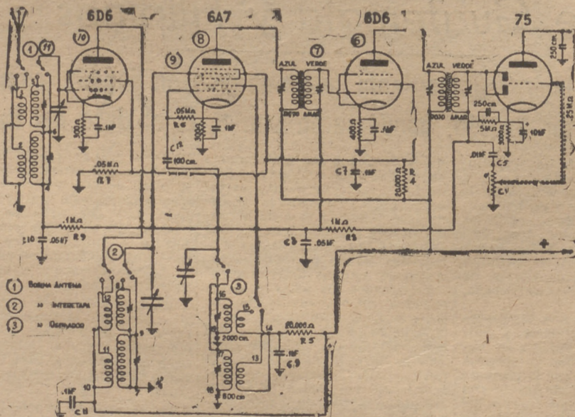
Figura 173.—Etapa de radiofrecuencia
