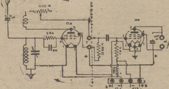
Fig. 107.—Esquema del receptor de una-dos lámparas
