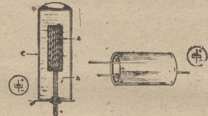
Fig. 19.—Corte de un condensador electrolítico con envoltura de aluminio. Fig. 20.—Condensador electrolítico doble, con envoltura de cartón.
