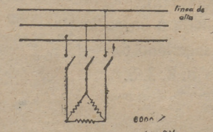
Esquema de instalación de un transformador triángulo-estrella
