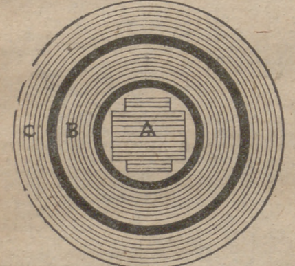
Sección de una rama de un transformador: A, núcleo; B, bobina de alta; C, bobina de baja.
