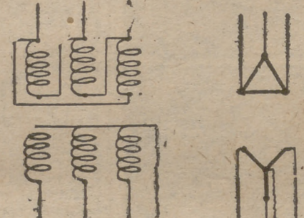
Dos esquemas representativos de transformador triángulo-estrella.
