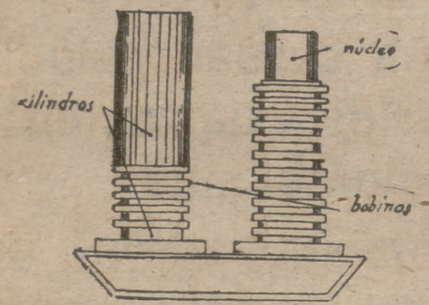
Detalle constructivo de un transformador monofásico.
