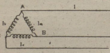
Unión de arrollamientos en triángulo
