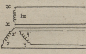
Unión de los arrollamientos (estrella)
