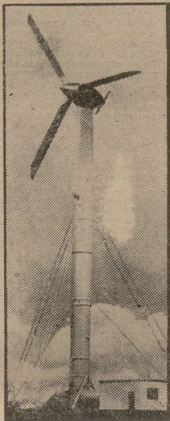
Modelo de aeroturbina que da lugar a una depresión en la columna de sostén de 150 kilovatios. Esta aeroturbina es de patente "Andreas". El paso variable y la puesta en bandera de las palas se consiguen automáticamente merced al pequeño molinete que se ve al extremo anterior del buje.
