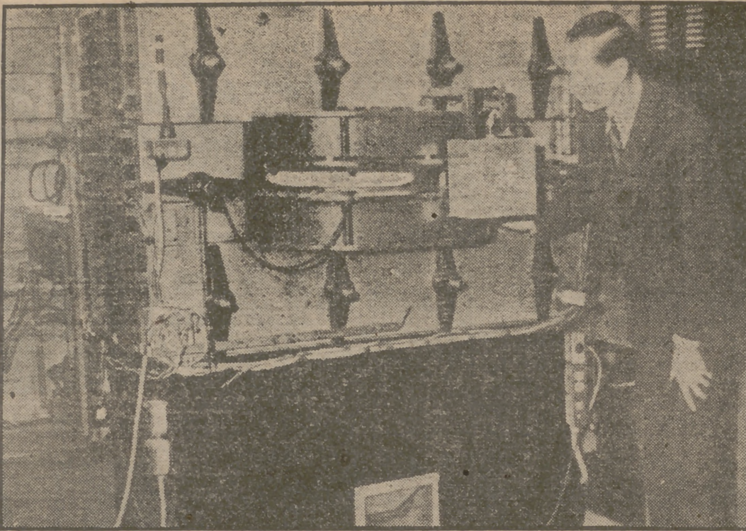
El doctor Donald W. Kerst, de la Universidad de Illinois, muestra su aparato de 25 millones de voltios Betatron, planteado y construido con la cooperación de la Universidad. Los científicos americanos esperan que la máquina abra formidables campos en la lucha contra el cáncer.
