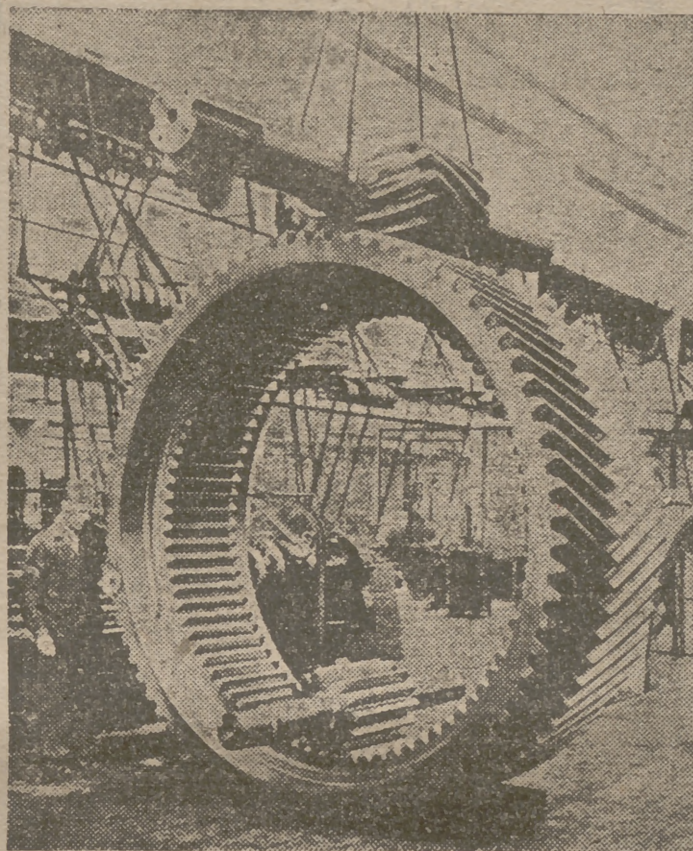
La fuerza impresionante de la industria se aprecia en la rotunda solidez de este gigantesco engranaje para máquinas laminadoras con corona forjada y piñones de acero, que pesa 23 toneladas.
