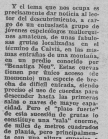
ALGUNAS «COLUMNAS» DE ESTA sala tienen más de treinta metros de altura. Entre las diversas formaciones calcáreas hay extrañas y sorprendentes formas que no tienen precedentes en ninguna de las cuevas conocidas y exploradas hasta el momento. Es de destacar la proliferación de los llamados «ranchos» —de los que existen sólo contadísimas muestras
