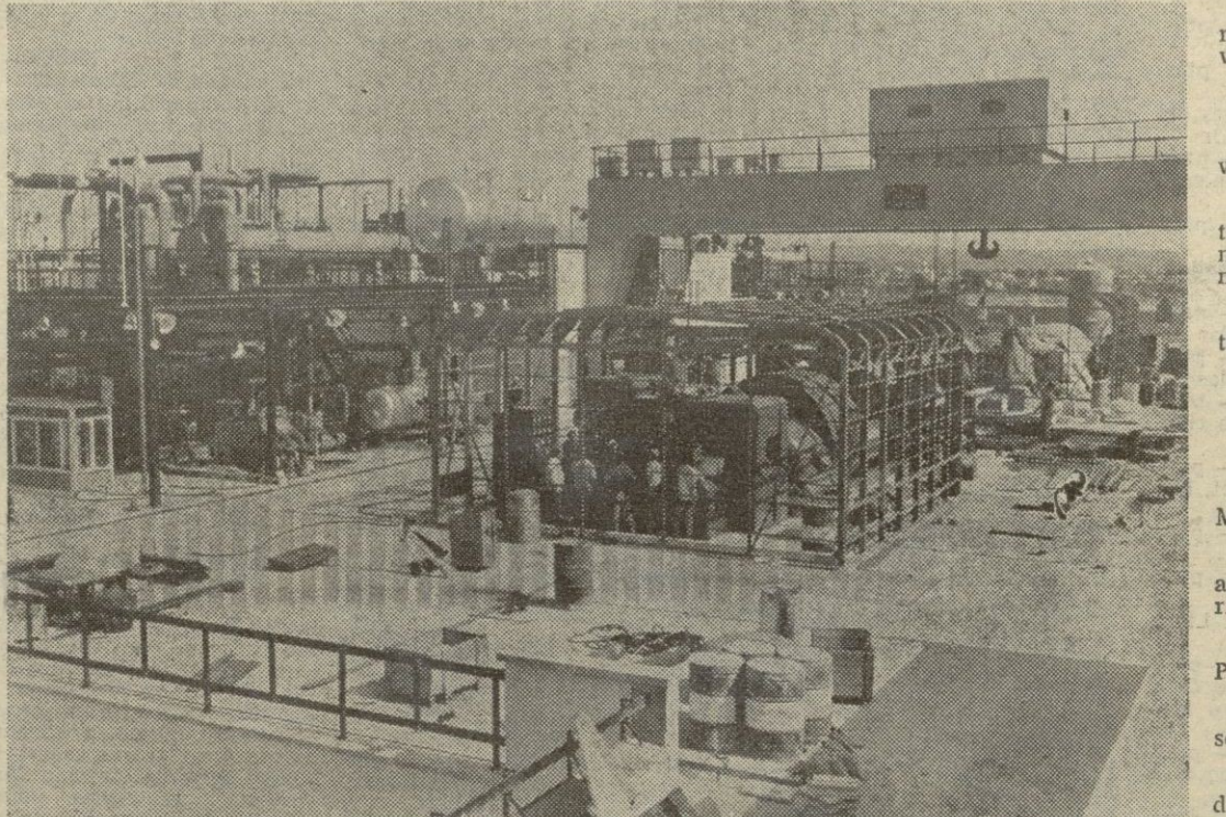
CENTRAL SAN JUAN DE DIOS (G.E. S.A.). - UN ASPECTO DEL MONTAJE.
