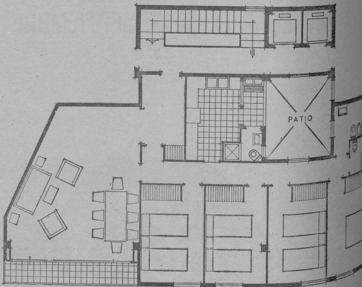
PLANTA PISO TIPO H
