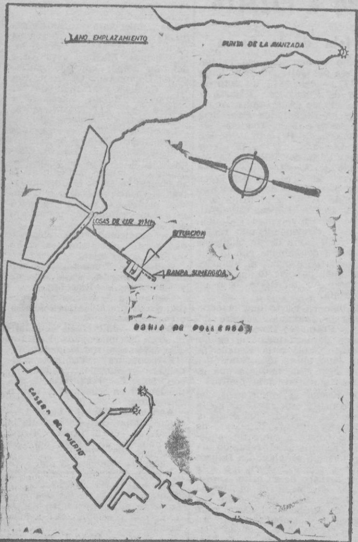
PLANO EN EL QUE PUEDE APRECIARSE LA SITUACION, FORMA Y LONGITUD DEL FUTURO MUELLE Y VARADERO. ES DE DESTACAR QUE EL EDIFICIO QUE FIGURA AL FINAL DEL MISMO, HA SIDO SUPRIMIDO POR NO SER AUTORIZADO.
