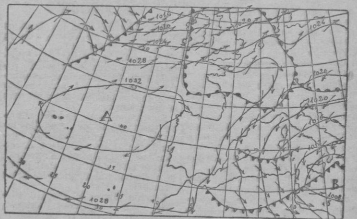
Situación atmosférica del día 3-II-62 a 06 h. T. M. G. (Facilitado por el Centro Meteorológico.)
