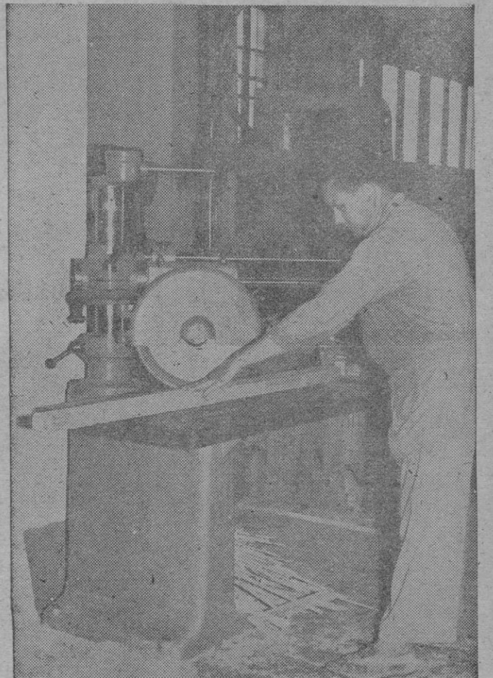
ESTA ES LA PRIMERA MAQUINA TRONZADORA RADICAL EXISTENTE EN LA ISLA
