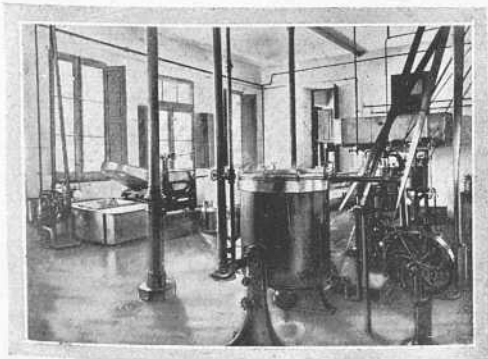
Sección de recepción, pasteurización y distribución de la leche.
