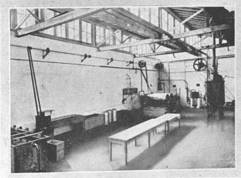
Sección de condensación y desecación.
