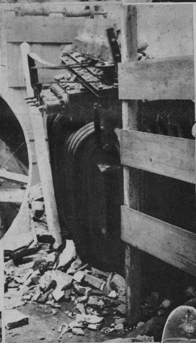
El transformador de la Metalgraf, destruido
