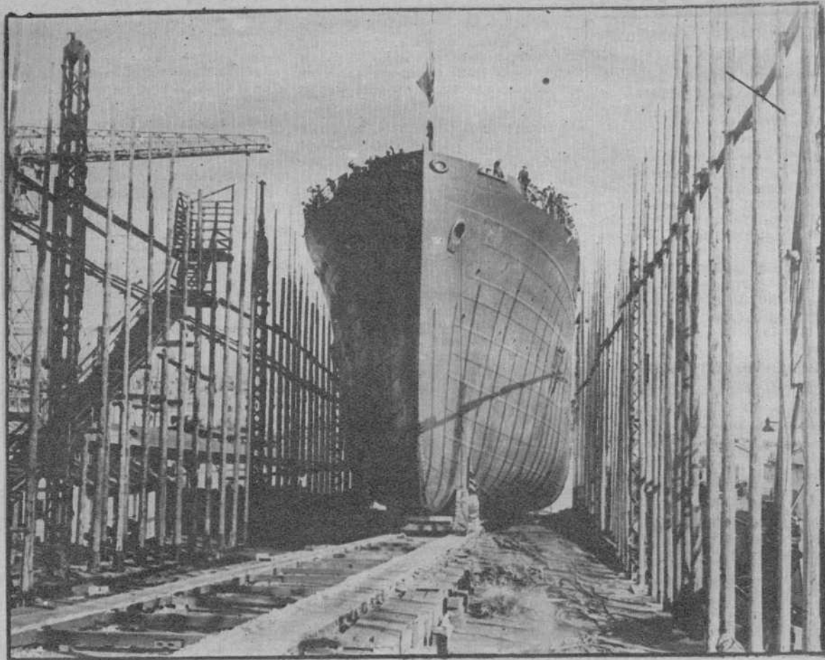
Marsella. — Botadura del nuevo buque francés «Presidente Paul Doumer»
