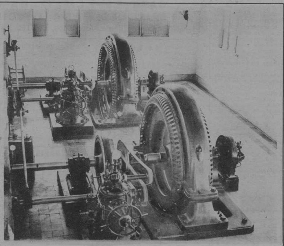
Interior de la sala de máquinas
