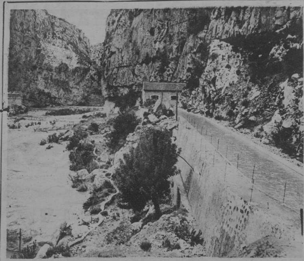
Tramo del Canal de conducción y casa de compuertas. En el estrecho del Río Turia, aguas arriba del pueblo de Chulilla.
