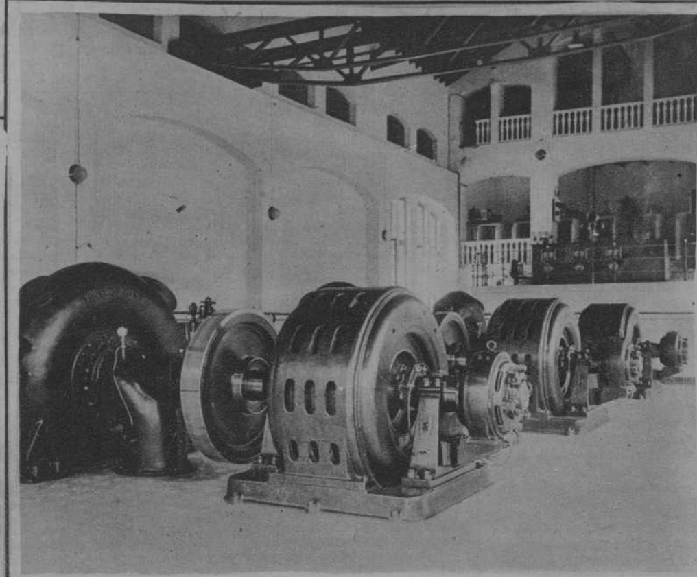
Interior de la sala de máquinas (3 grupos de 1.200 KVA cada uno)
