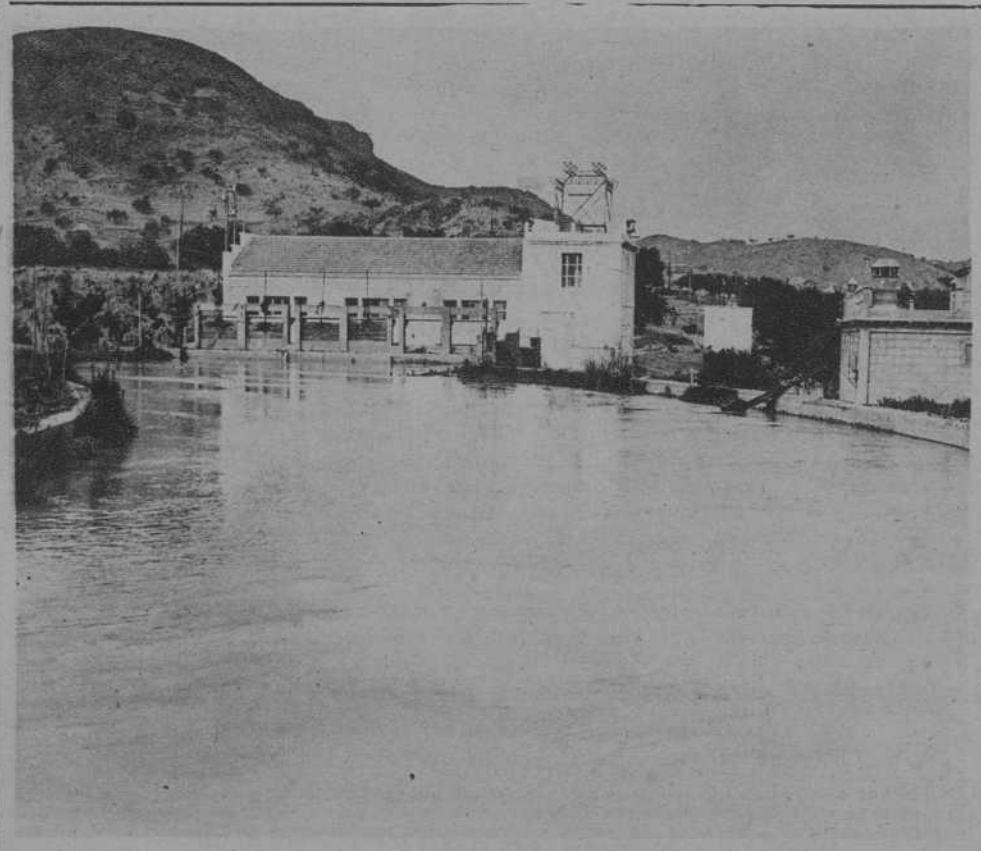
Cámara de carga y central
