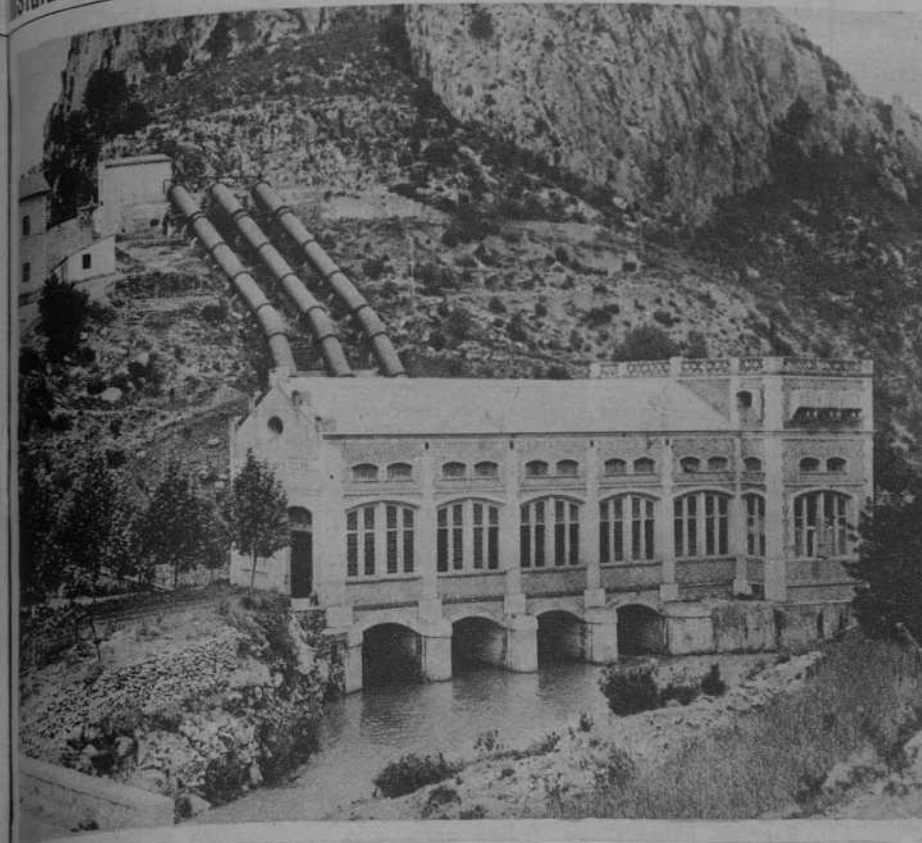
Cámara de carga, tubería de presión, central y canal de desagüe
