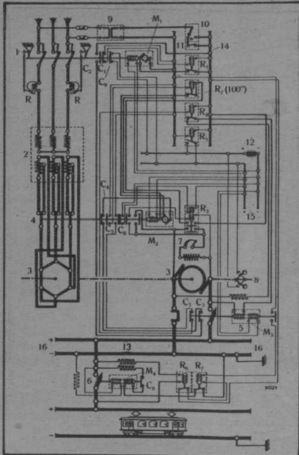
Fig. 2. Esquema de una estación automática de transformación
