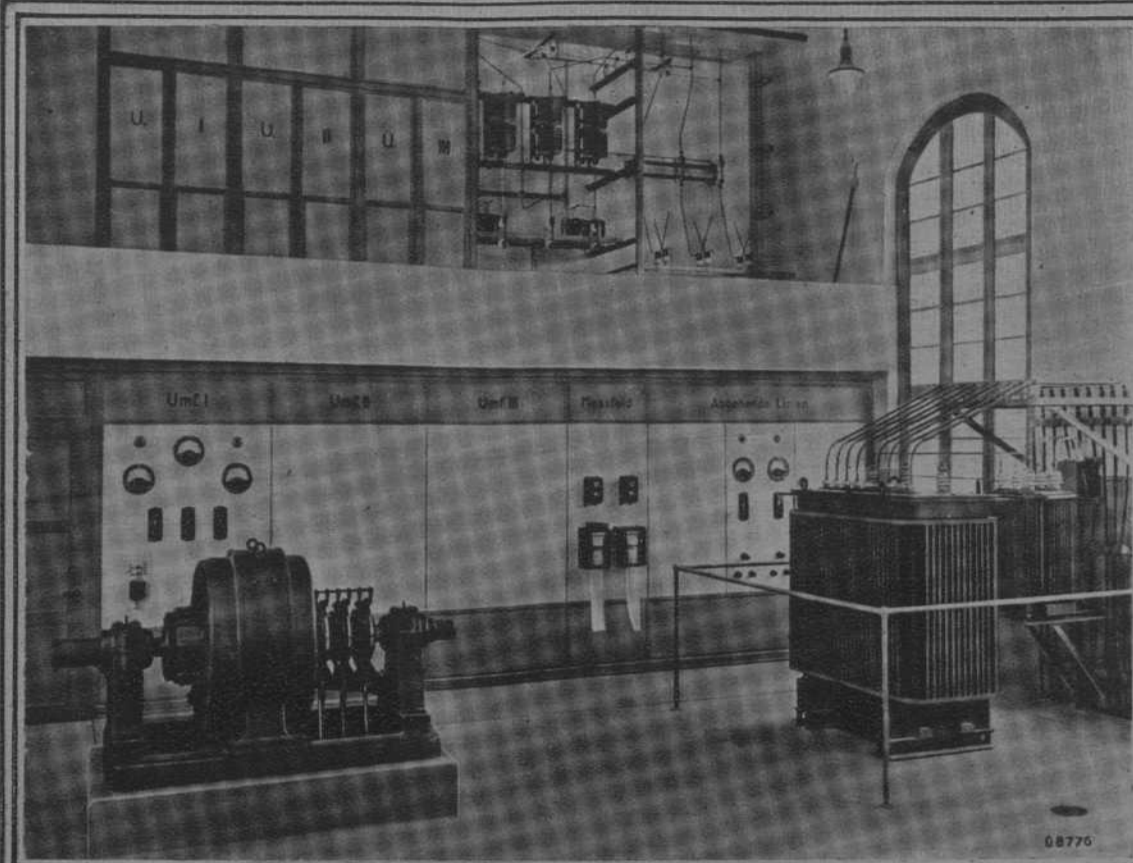
Fig. 1. Sala de máquinas y cuadro de distribución de la estación automática de transformación de Riehen (Basilea).
