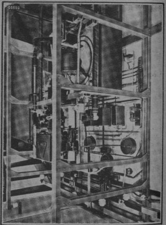
Fig. 3. Vista del panel de la conmutatriz desde el lado posterior.
