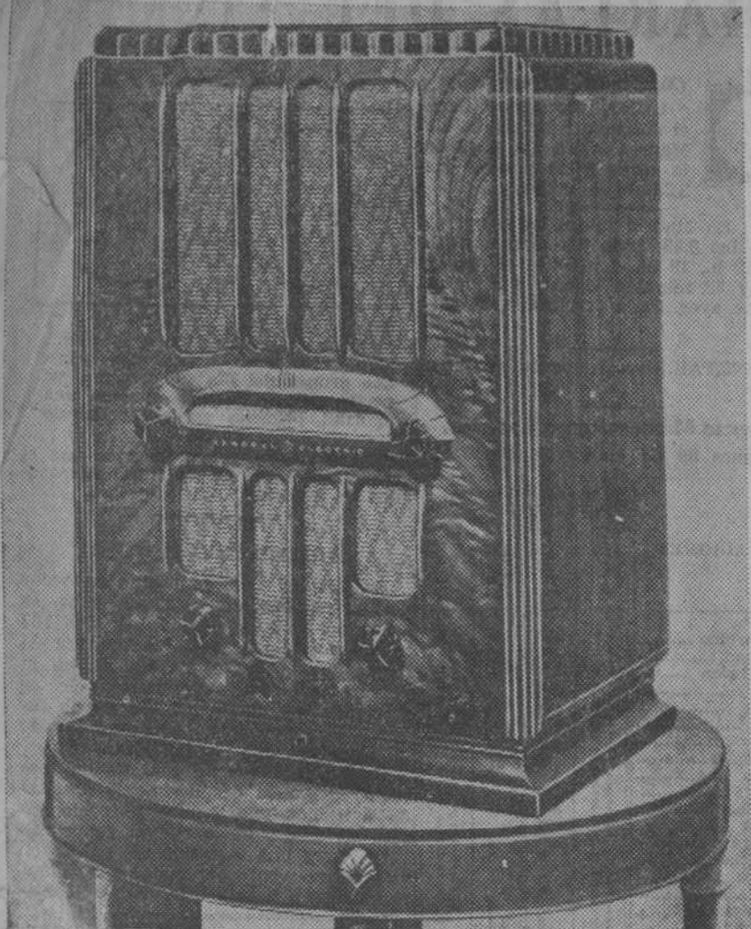
Modelo A-70 General Electric. Aparato de sobremesa para cuatro bandas, cubriendo todas las estaciones de onda larga y normal, así como las de frecuencias extraortras. Equipado totalmente con válvulas metálicas. La caja ofrece una agradable y modernista apariencia. Presentado por S. I. C. E.
