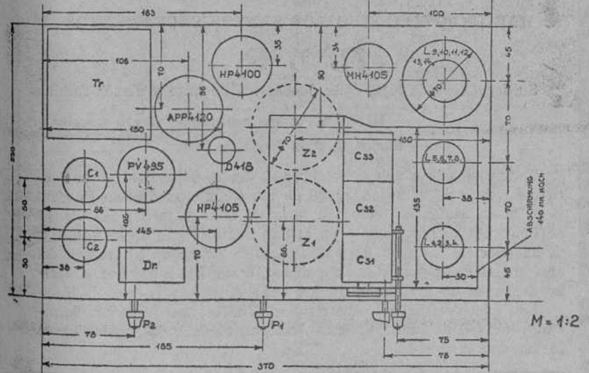
Publicamos la explicación del esquema Tungsram para superheterodino de 6 válvulas por corriente alterna, todas ondas, publicado en nuestra página del 19 del pasado mes. En la próxima publicaremos la lista de materiales.
