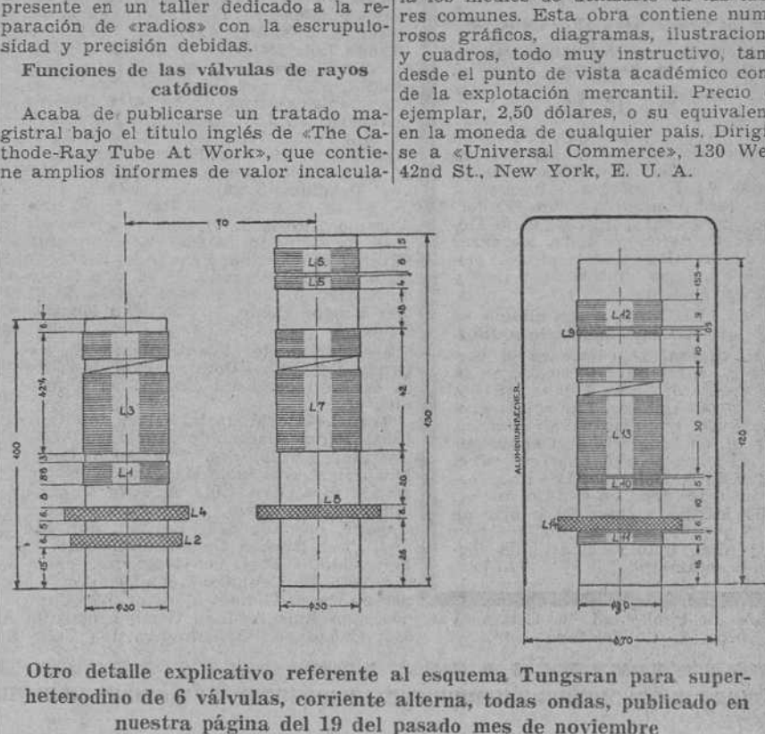
Otro detalle explicativo referente al esquema Tungsram para superheterodino de 6 válvulas, corriente alterna, todas ondas, publicado en nuestra página del 19 del pasado mes de noviembre
