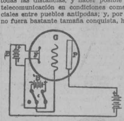
Figura 1. Triodo de Lee de Forest
