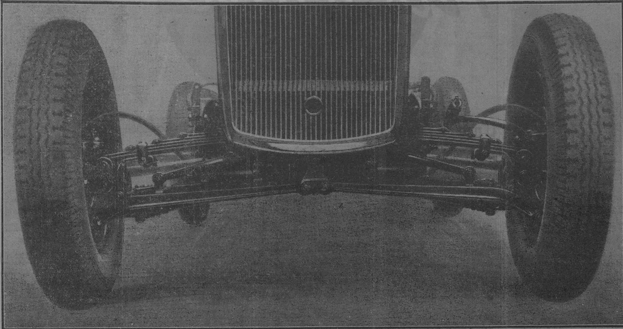
Sustituido el eje rígido de las ruedas delanteras por unos brazos y resortes articulados, cada una de las ruedas vence baches y pedruscos y pequeños obstáculos, sin que el coche sufra saltos y bandazos
