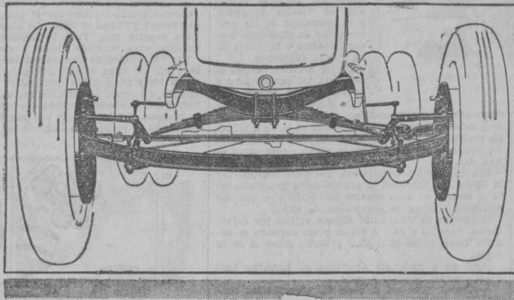
Nuevos ejes y ballesta delanteros.
