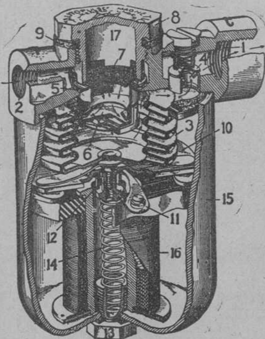
Corte seccional del nuevo auto-propulsor magnético.
