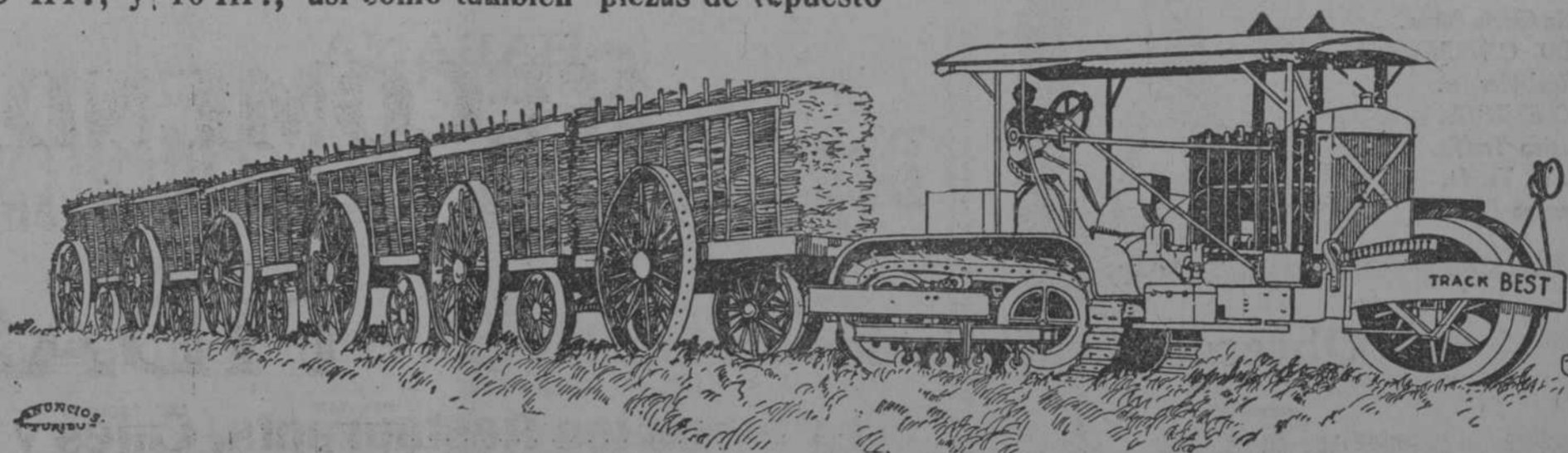
Tractor "TRACKLAYER", de 75 HP., tirando 6 carros de caña, en la finca Santa Ana, del Señor Juan Maa, de Sagua la Grande
