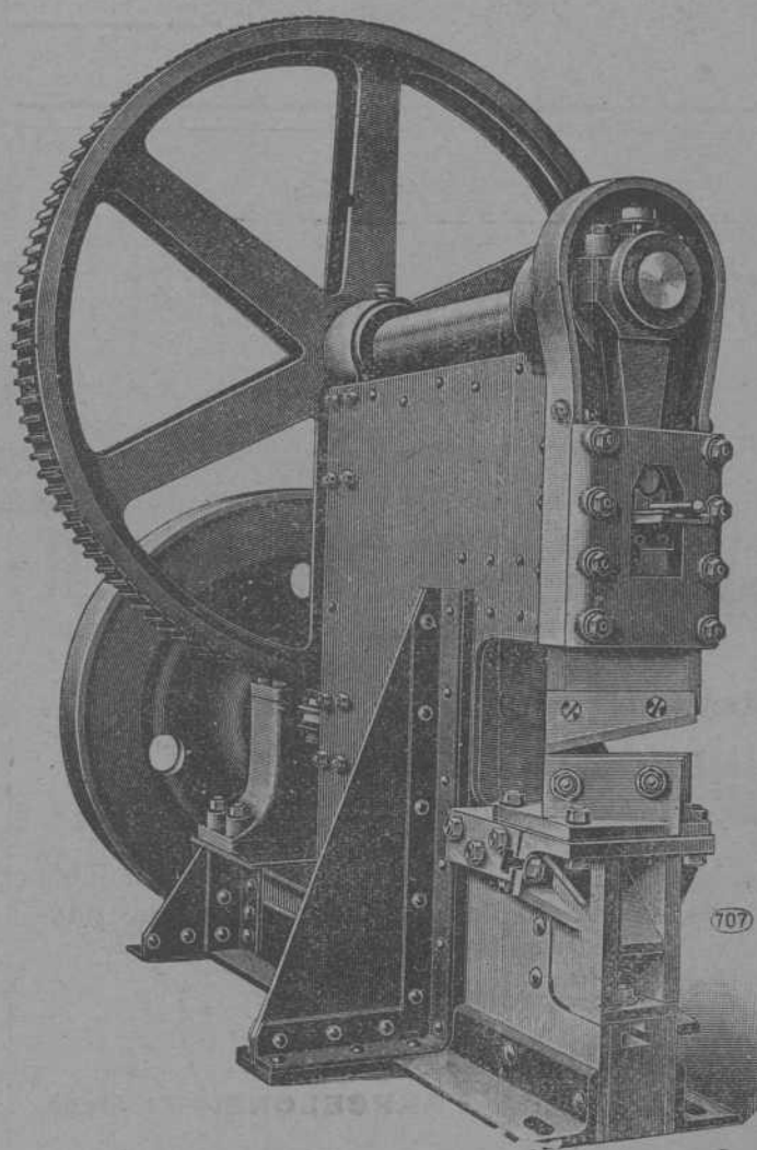
LA MISMA MÁQUINA COMO CIZALLA PARA CORTAR PLANCHAS
