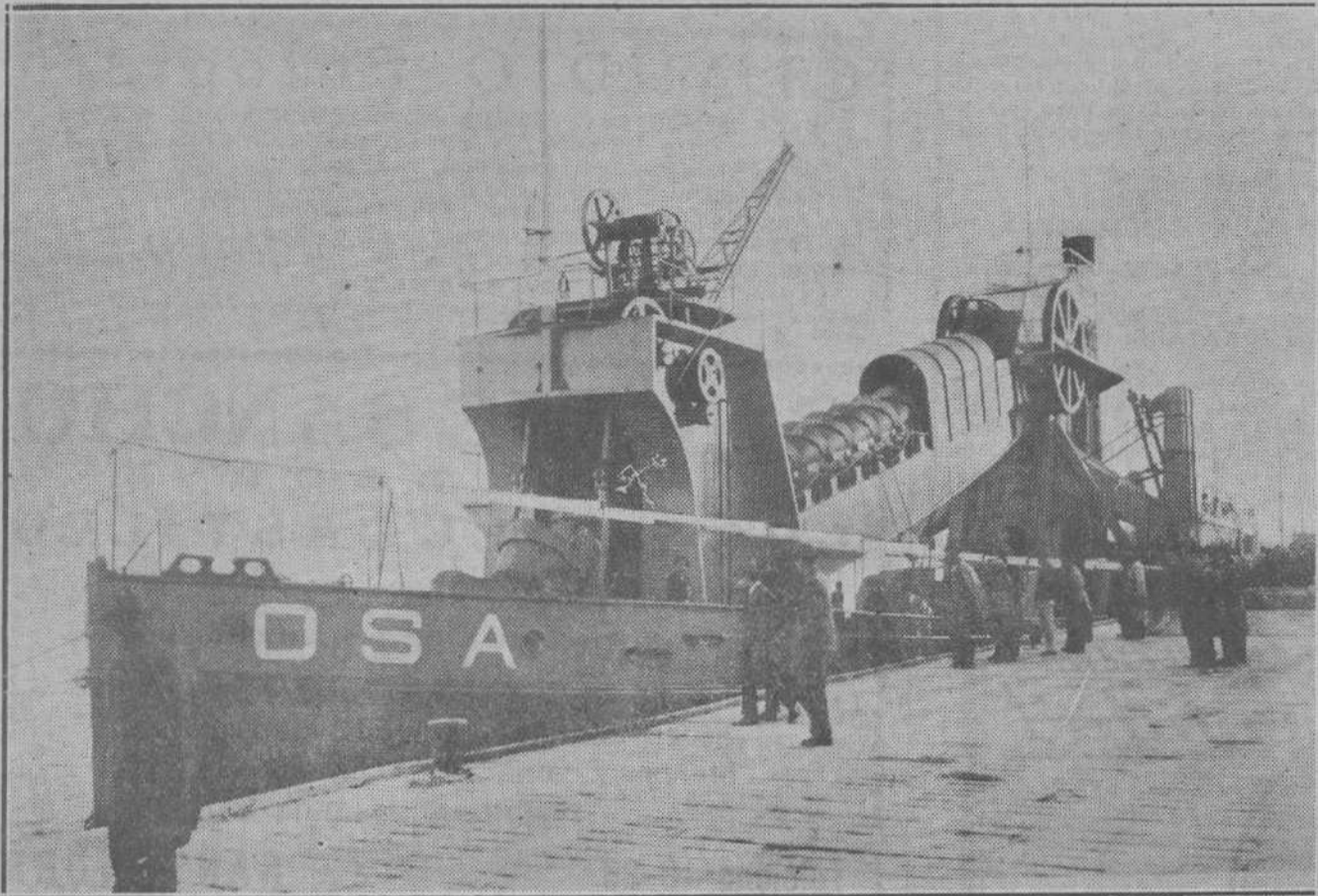
La nueva y magnífica draga, adquirida por la Junta de Obras del Puerto, y que ayer llegó a Santander. (Foto Alejandro.)
