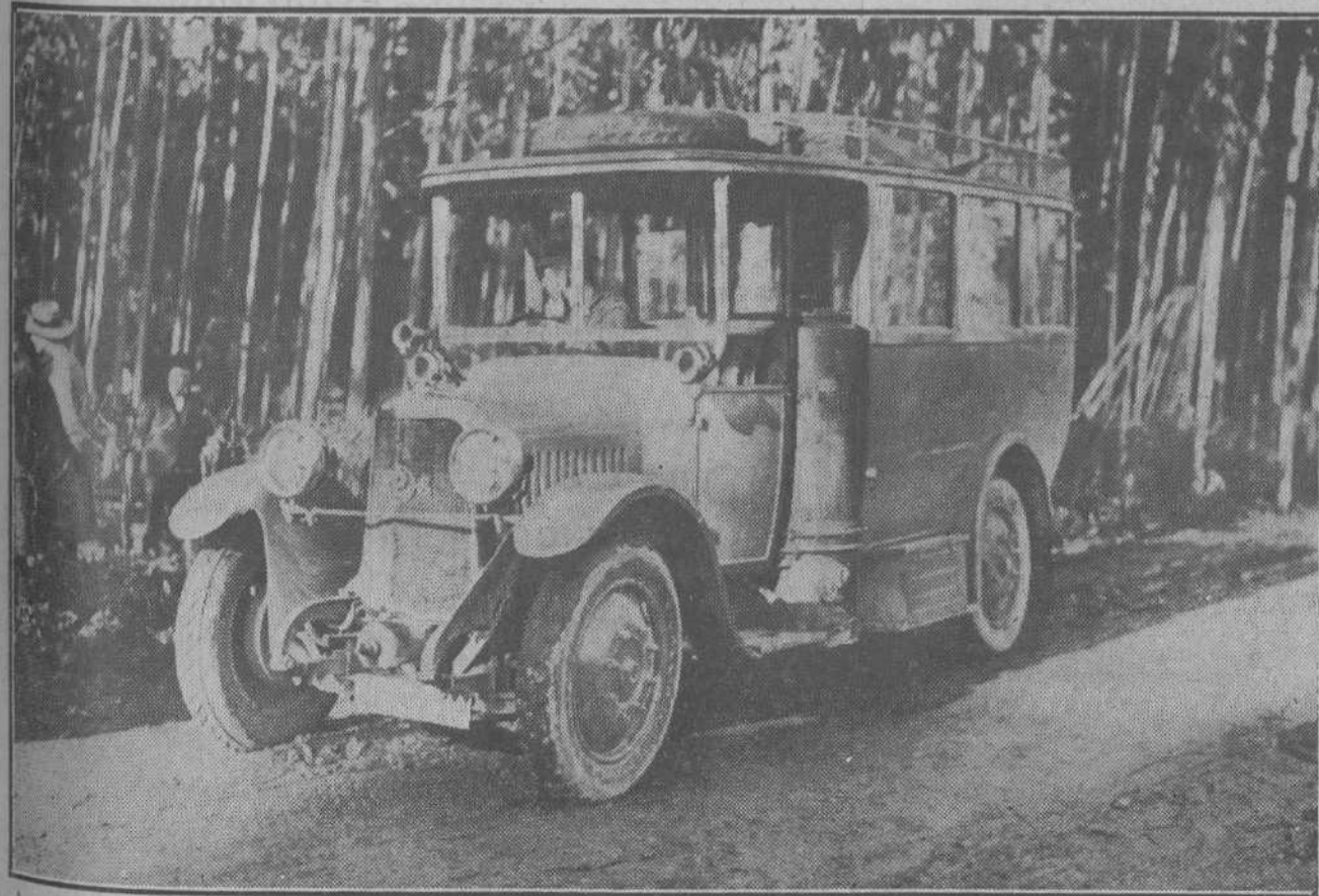
DE UNAS INTERESANTES EXPERIENCIAS.—El automóvil movido por gas de carbón, en sustitución de gasolina, que trajo a sus órdenes el ingeniero señor Bernard como una prueba interesantísima de los de esta naturaleza que se realizarán en breve en Torrelavega. (Fotos Alejandro).
