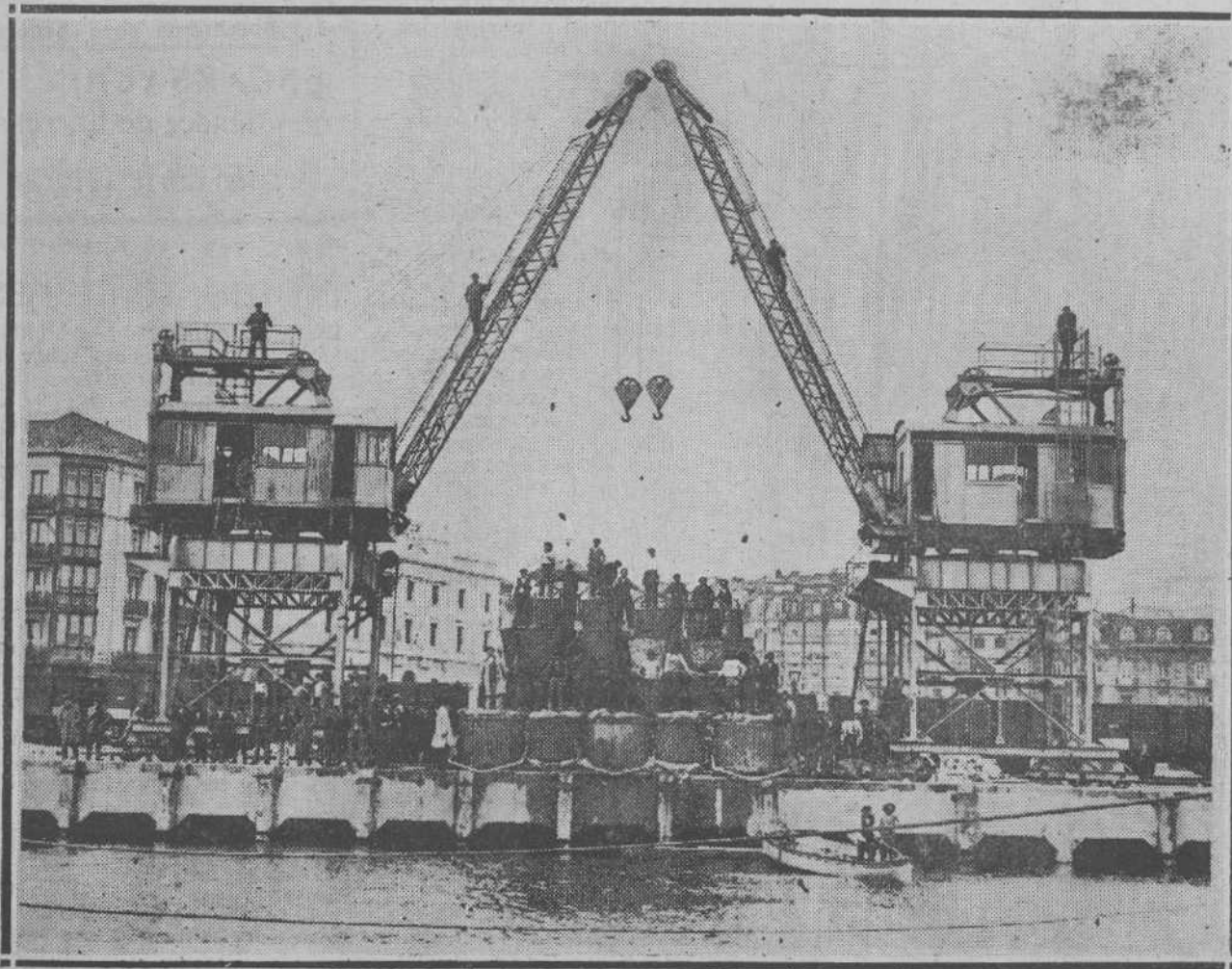
Este grabado representa las últimas pruebas de resistencia en los nuevos muelles de cemento. En el de Albareda se hicieron estas pruebas estáticas con una carga de ciento noventa mil kilos, a base de arena y rieles.
