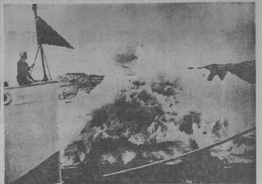
El análisis de los profundos núcleos de hielo existentes en Groenlandia permite afirmar a los científicos que cada vez hará más frío. (Foto Efo).
