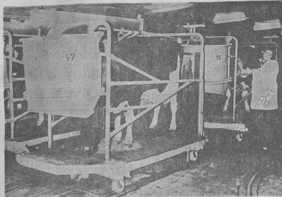
En Alemania Occidental la ganadería es objeto de la preferente atención de los técnicos. Ahora está investigándose un procedimiento para alimentar y ordeñar 60 vacas en una hora. Es un establo con jaulas sobre ruedas y un sistema automático de ordeño, obteniéndose mejor calidad de la leche, animales más sanos y menor trabajo para el granjero.
