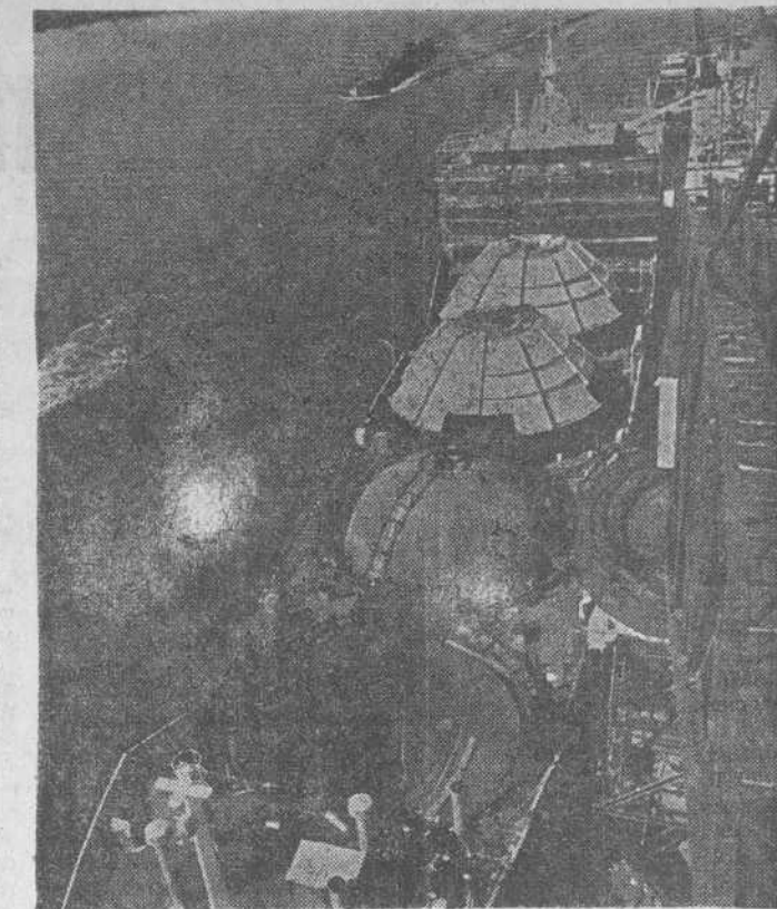
El grupo francés «Gazocean» ha puesto en servicio en el Atlántico, entre Argelia y Estados Unidos, este buque cisterna, el «Eucledes», con recipientes esféricos de acero al 9 por 100 de níquel, cada uno con una capacidad de mil metros cúbicos de gas natural licuado.
