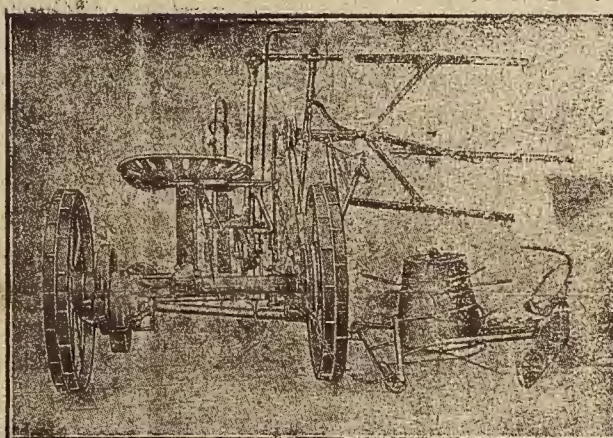
Guadañadoras con Molinete (Merveilleux). Para dejar el alfalfa en hilera.
