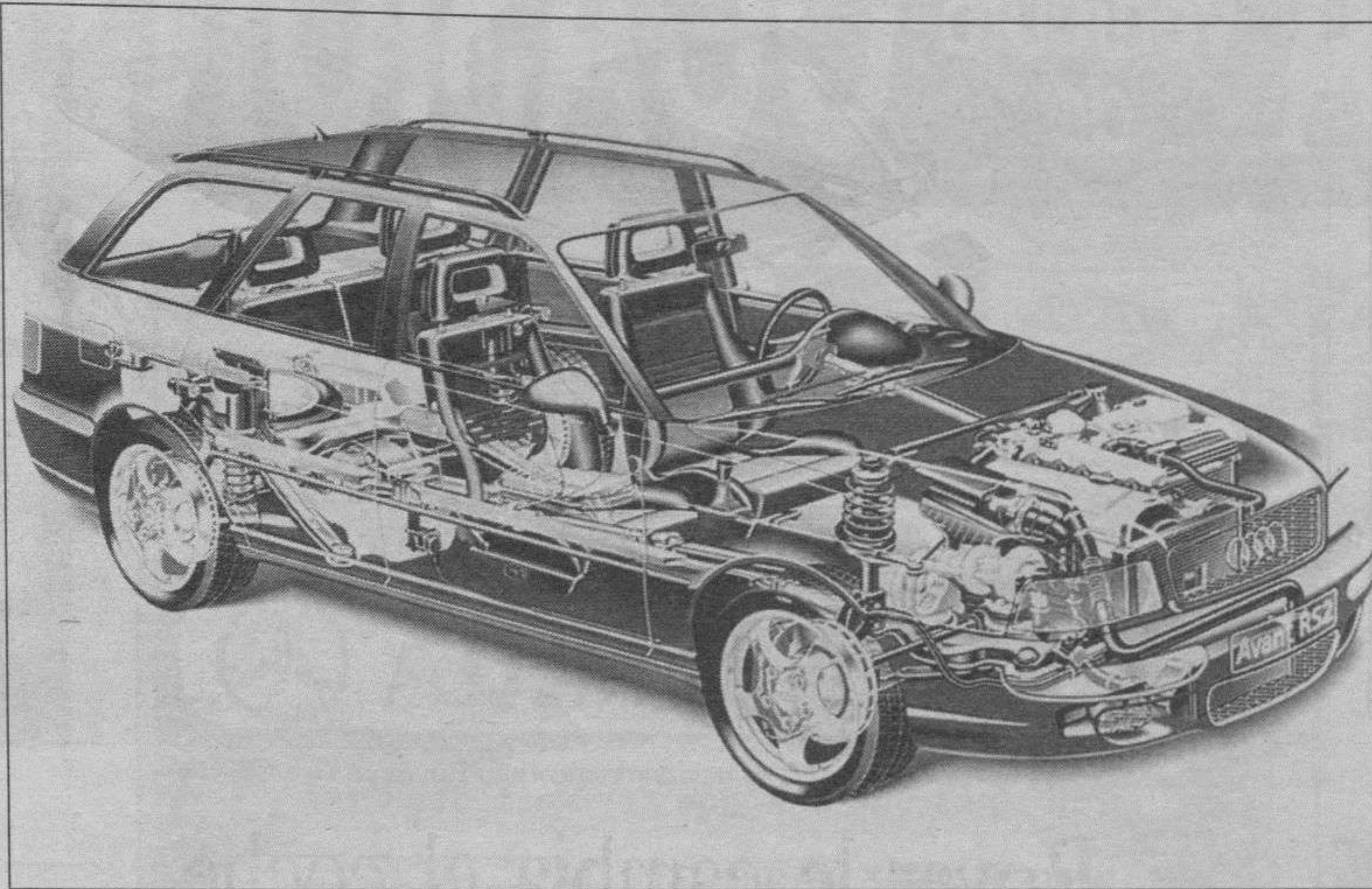
Motor, tracción, suspensiones, frenos y chasis de carreras en una carrocería poco habitual
