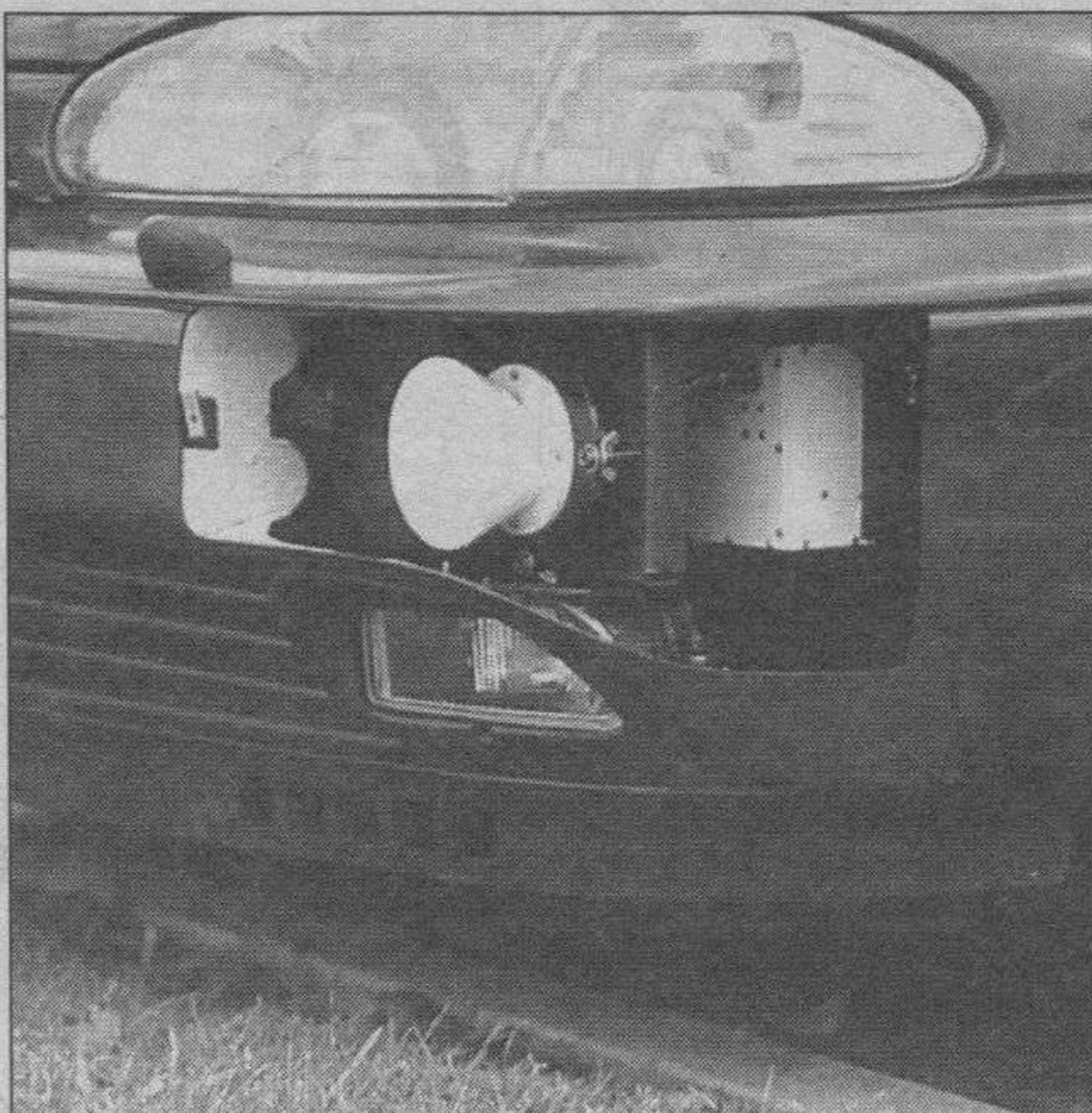
Radar para el control de velocidad, en el paragolpes
