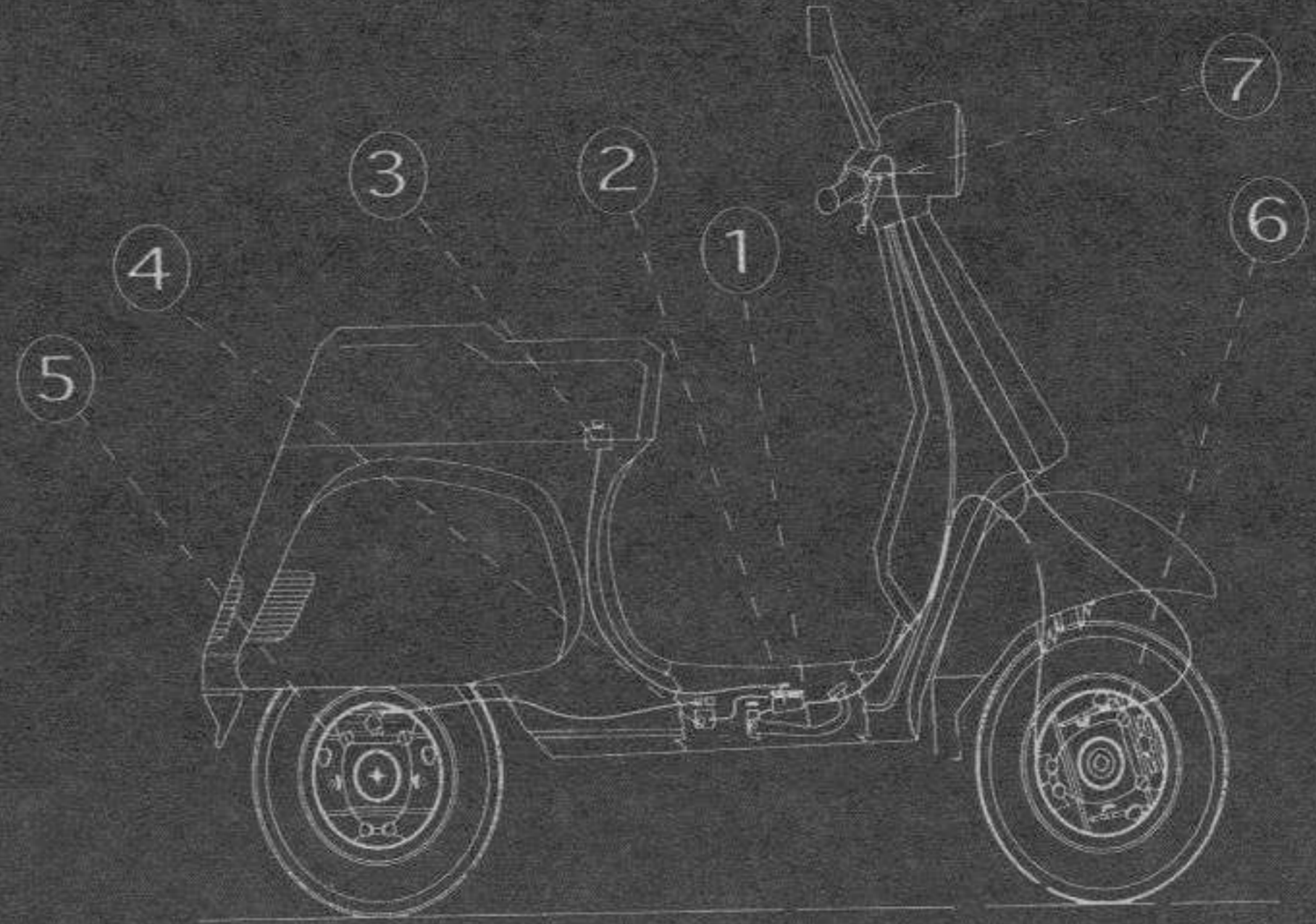
1- Pedal de freno; 2- Unidad de Control Hidráulico (HCU); 3- Depósito de líquido de frenos; 4- Unidad de Control Electrónico (ECU); 5- Válvula de regulación de Hidráulico; 6- Sensor de velocidad; 7- Maneta del freno delantero.
