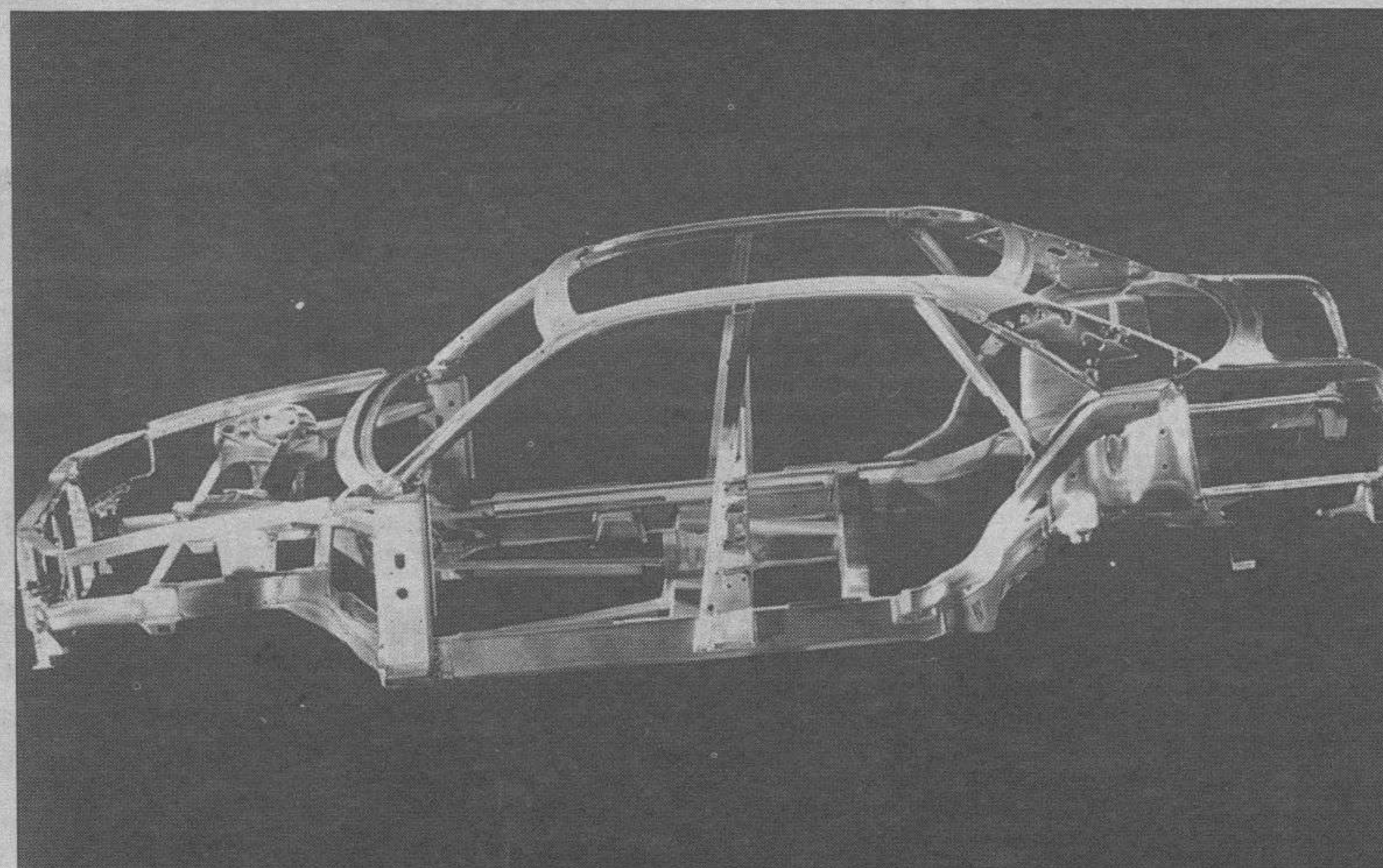
La estructura del bastidor se forma por perfiles extrusionados rectos y curvos muy resistentes.
