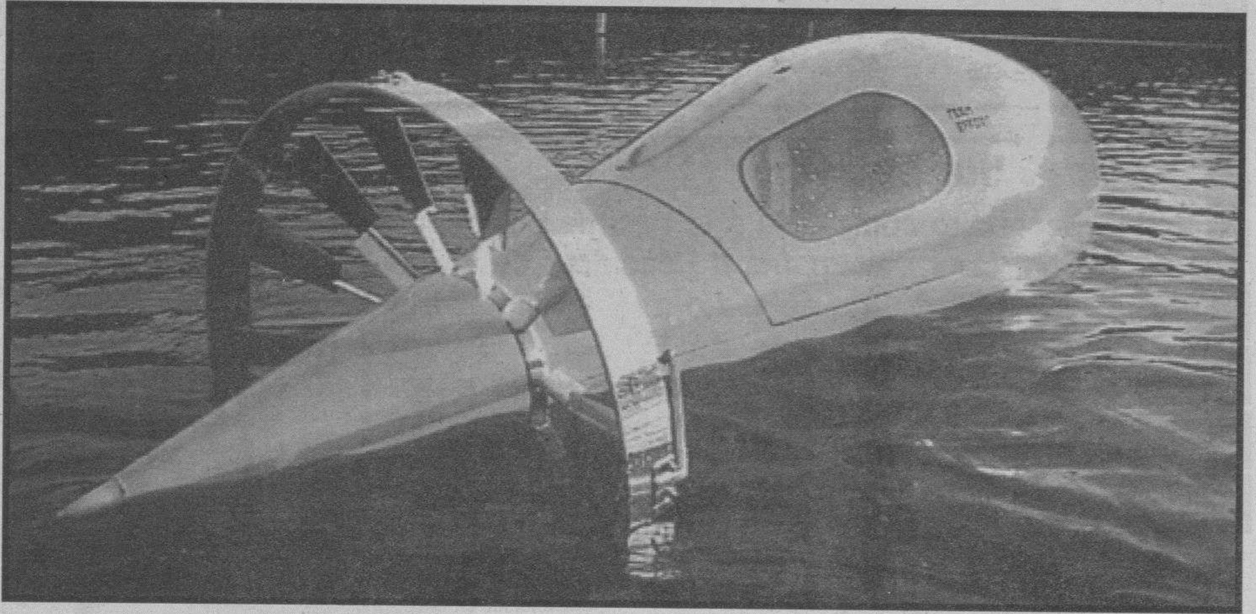
Submarinos con hélice en corona
