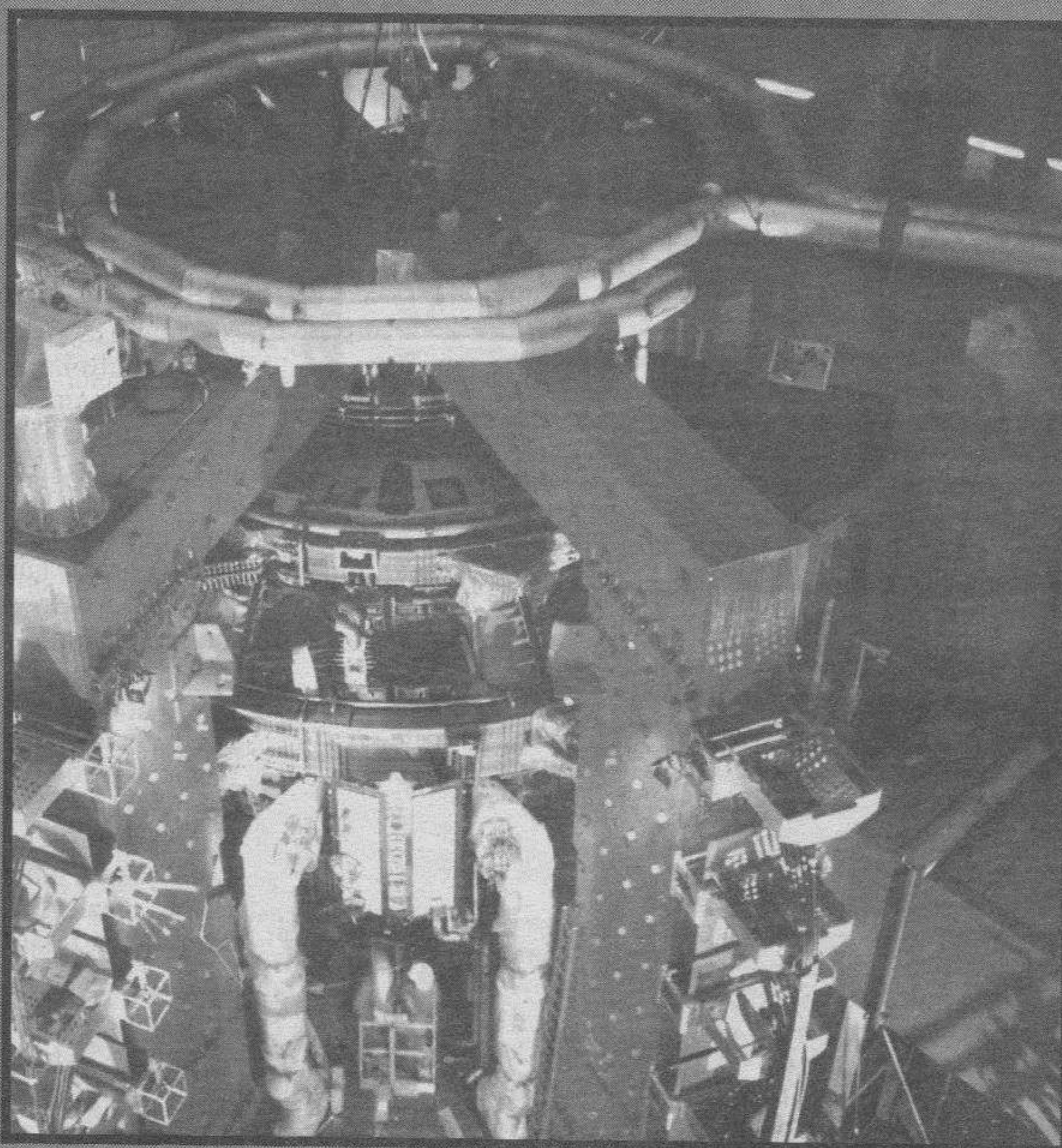
En las entrañas del JET (Joint European Torus) se produjo el prodigio, durante dos segundos, de la primera experiencia de fusión controlada.
