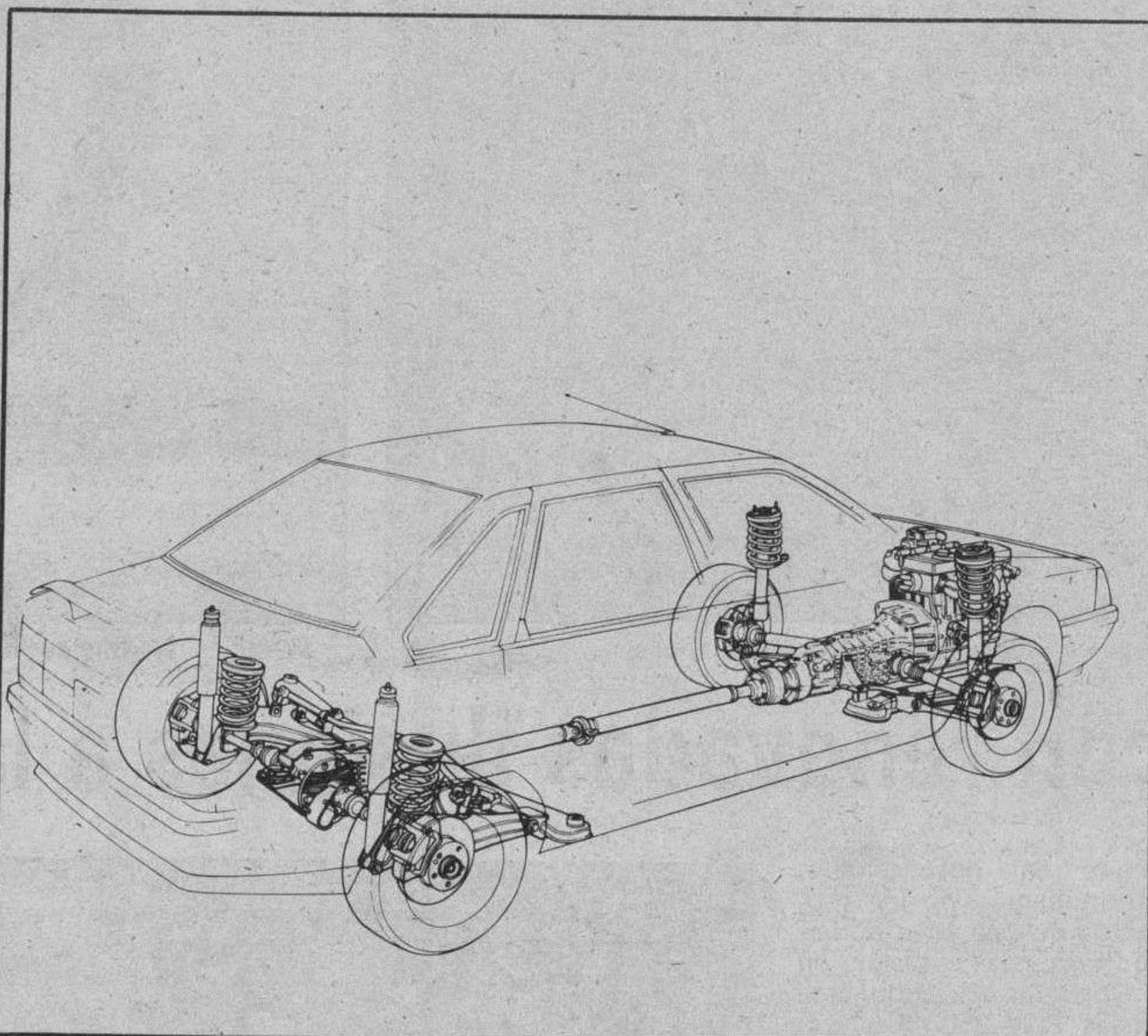
Radiografía de la transmisión total del Renault 21 TXI 4x4
