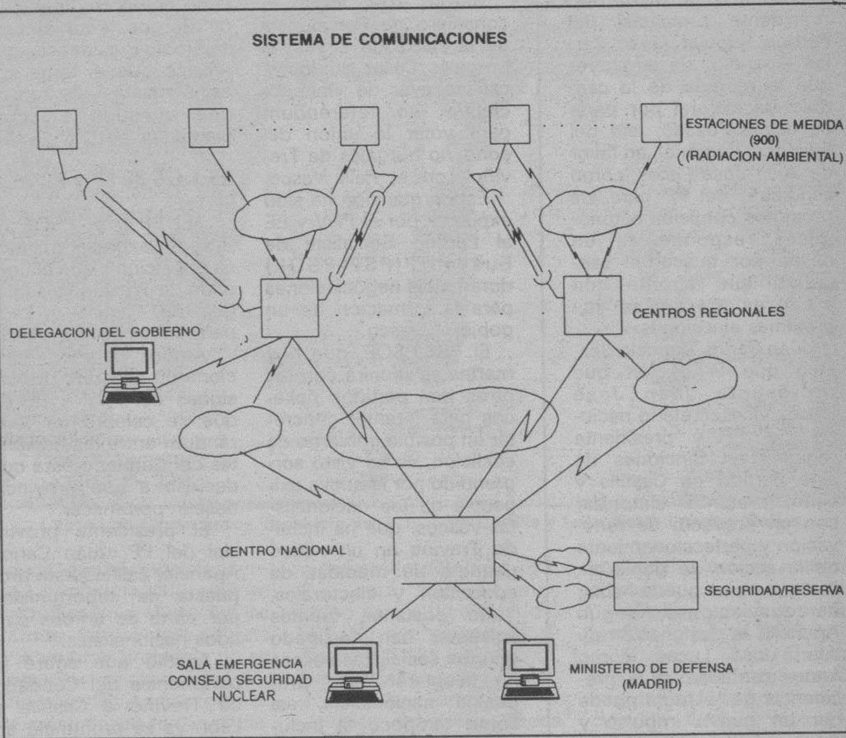
Sistema de comunicaciones previsto por la Dirección General de Protección Civil (De la revista Protección Civil)
