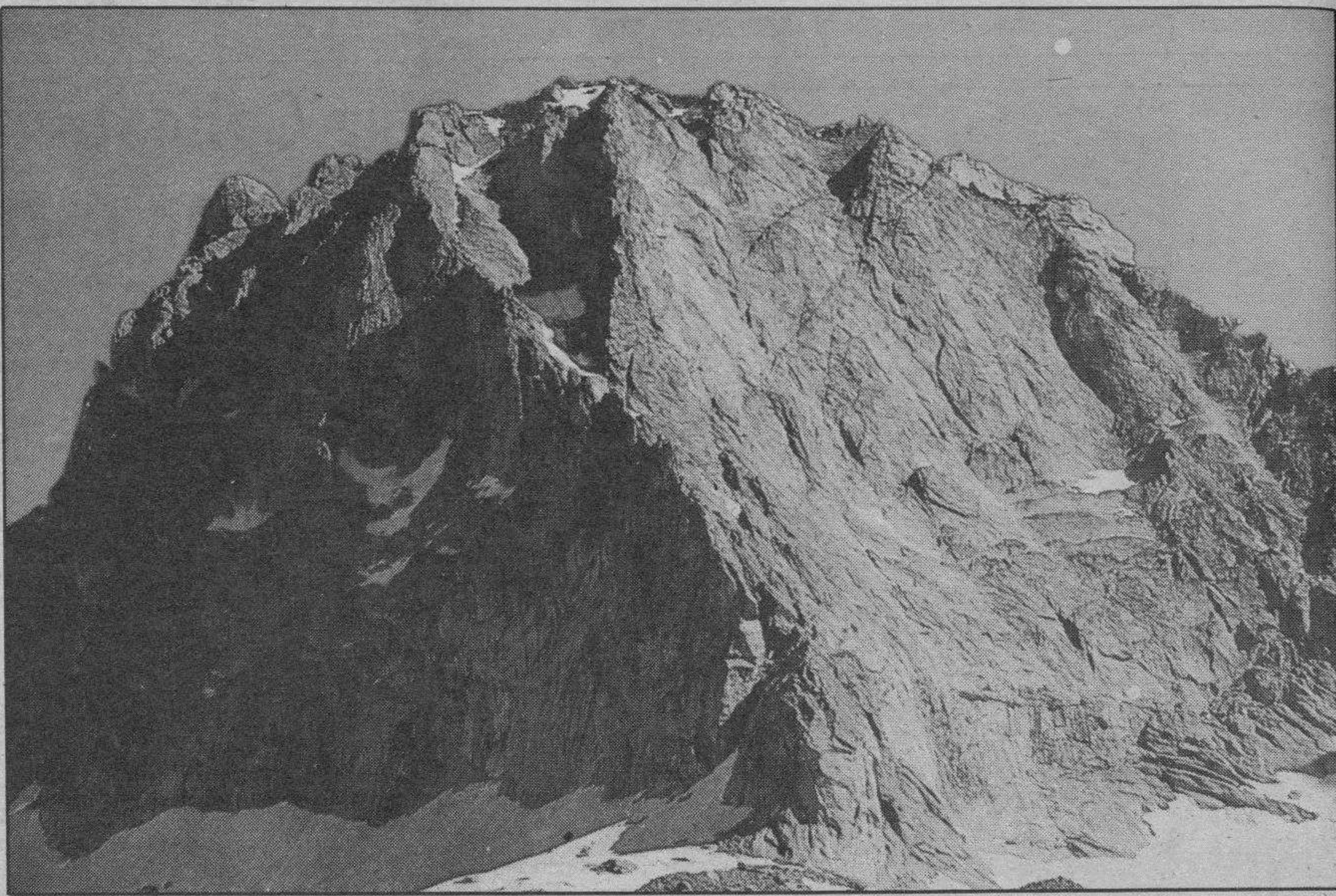
Cara S.O. del Piz Badile por donde discurre su ruta normal.
