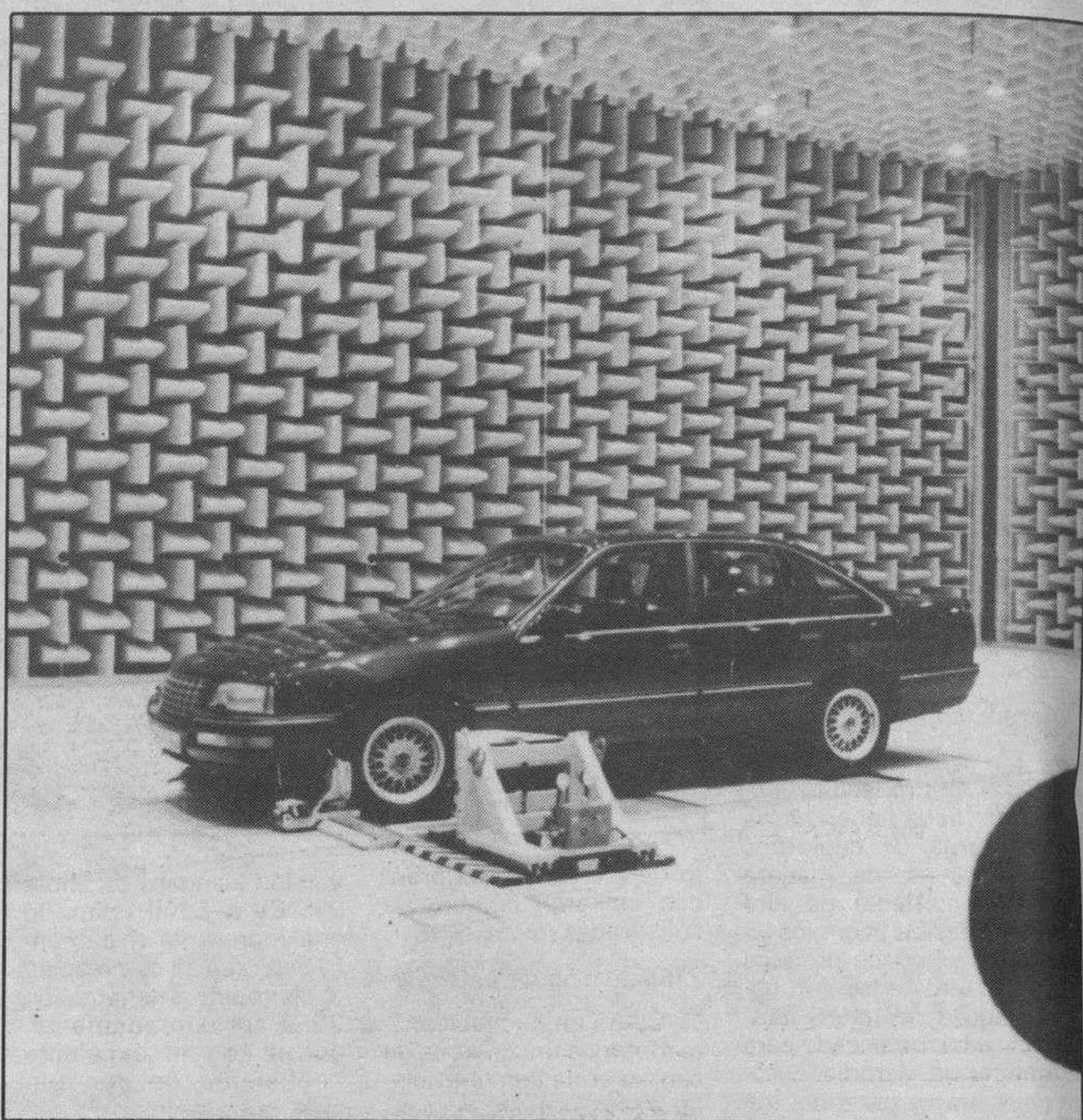
Opel investiga sobre el ruido en un banco de pruebas controlado por ordenador
