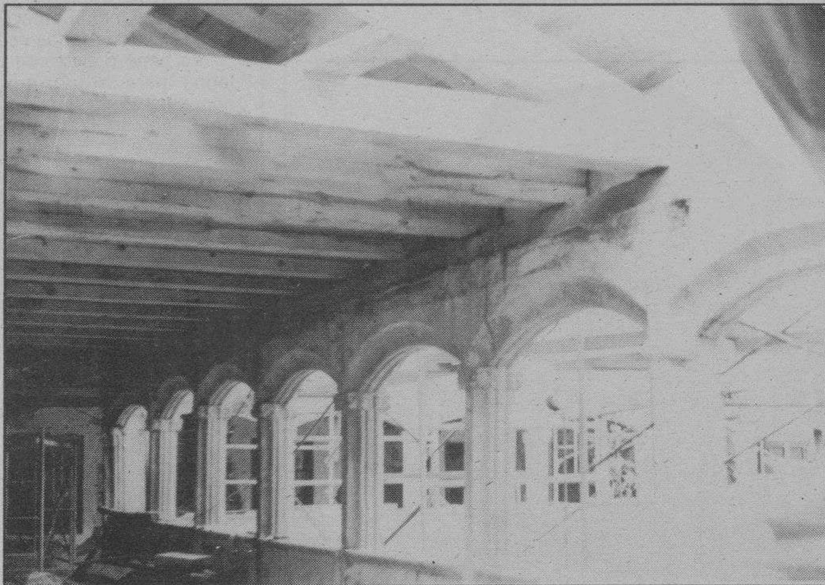
Parte superior del claustro. Retirada la techumbre, la fotografía nos señala las nuevas viguetas de madera que soportarán el nuevo techo.
