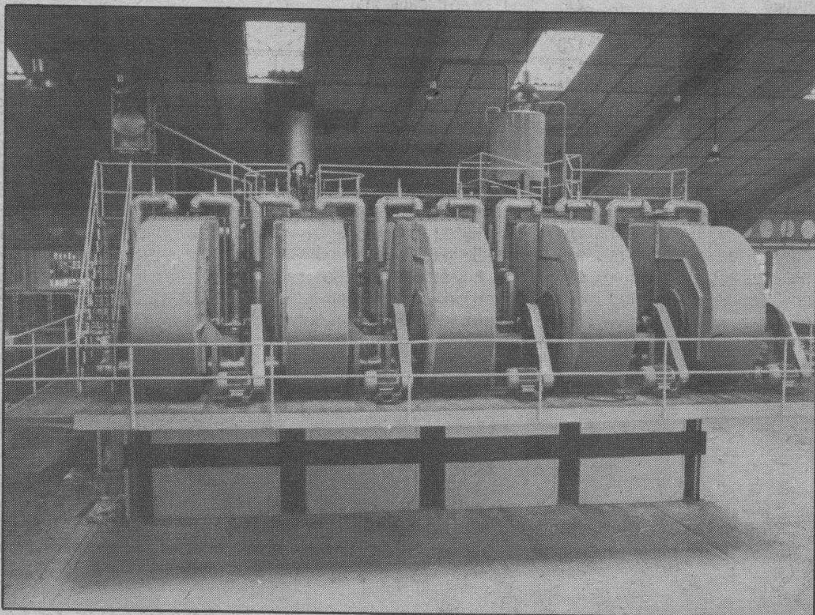
Túneles de secado, donde las colas se colocan en perfectas hileras, con el fin de dejar pasar el aire
