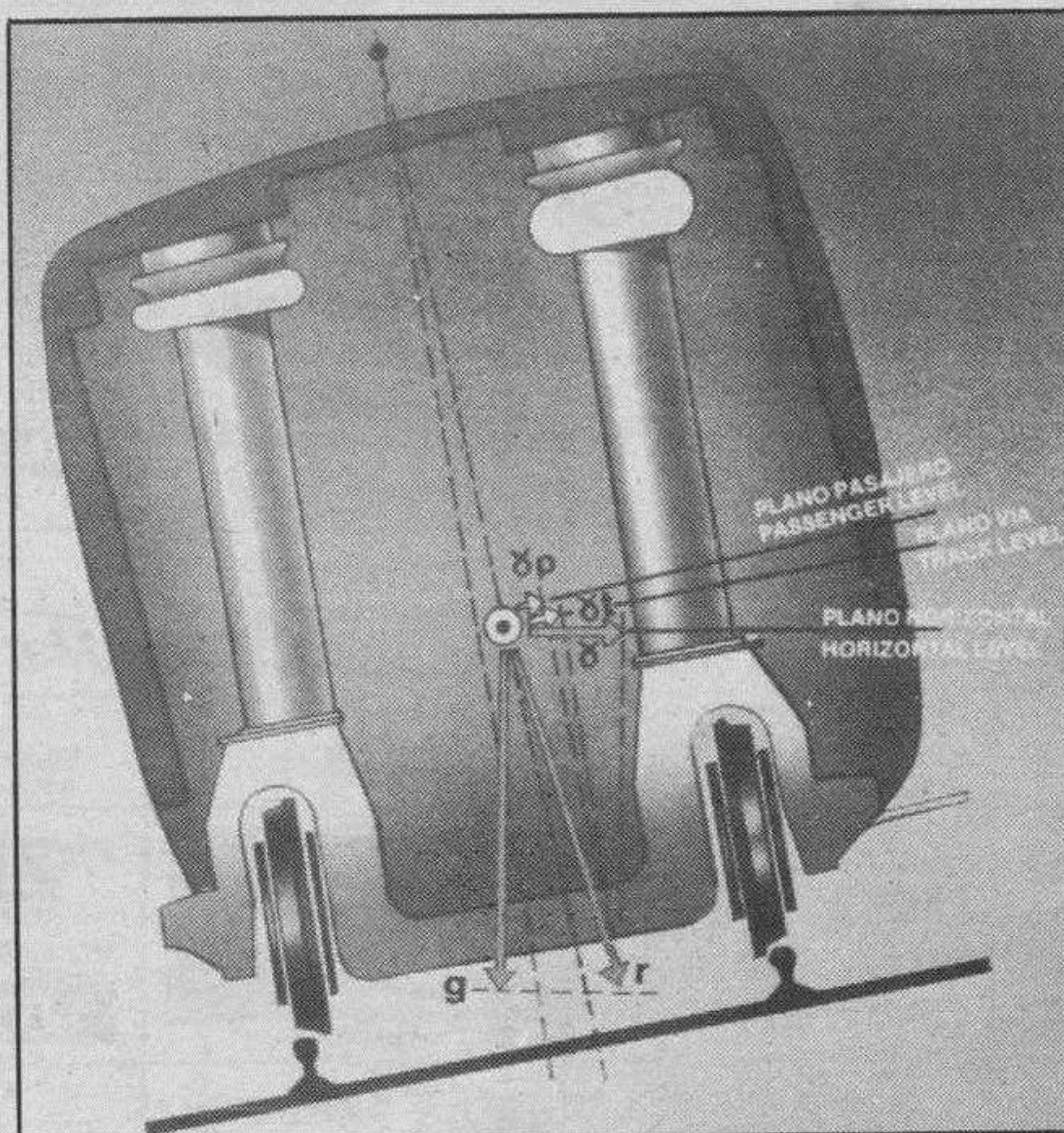
El sistema de pendulación natural se basa en elevar el plano de la suspensión muy por encima del centro de gravedad del coche. Foto Efe.
