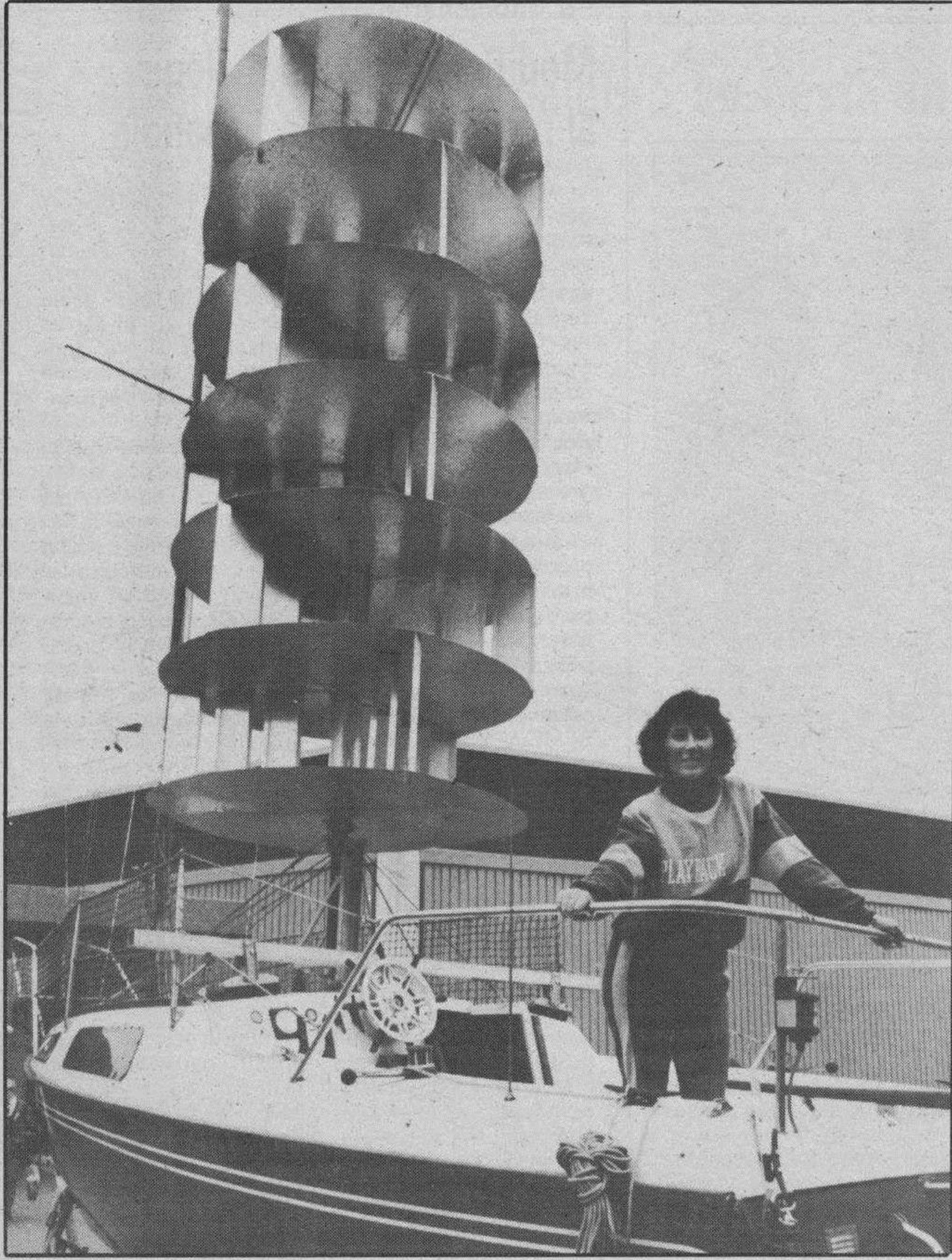
Feria de inventores. — El rotor eólico vertical «Wiwian» precisa apenas viento para impulsar la lancha a través de una hélice de barco acoplada. Este generador eólico es una de las muchas novedades presentadas a la feria internacional de inventores «INEA», de Nuremberg.
