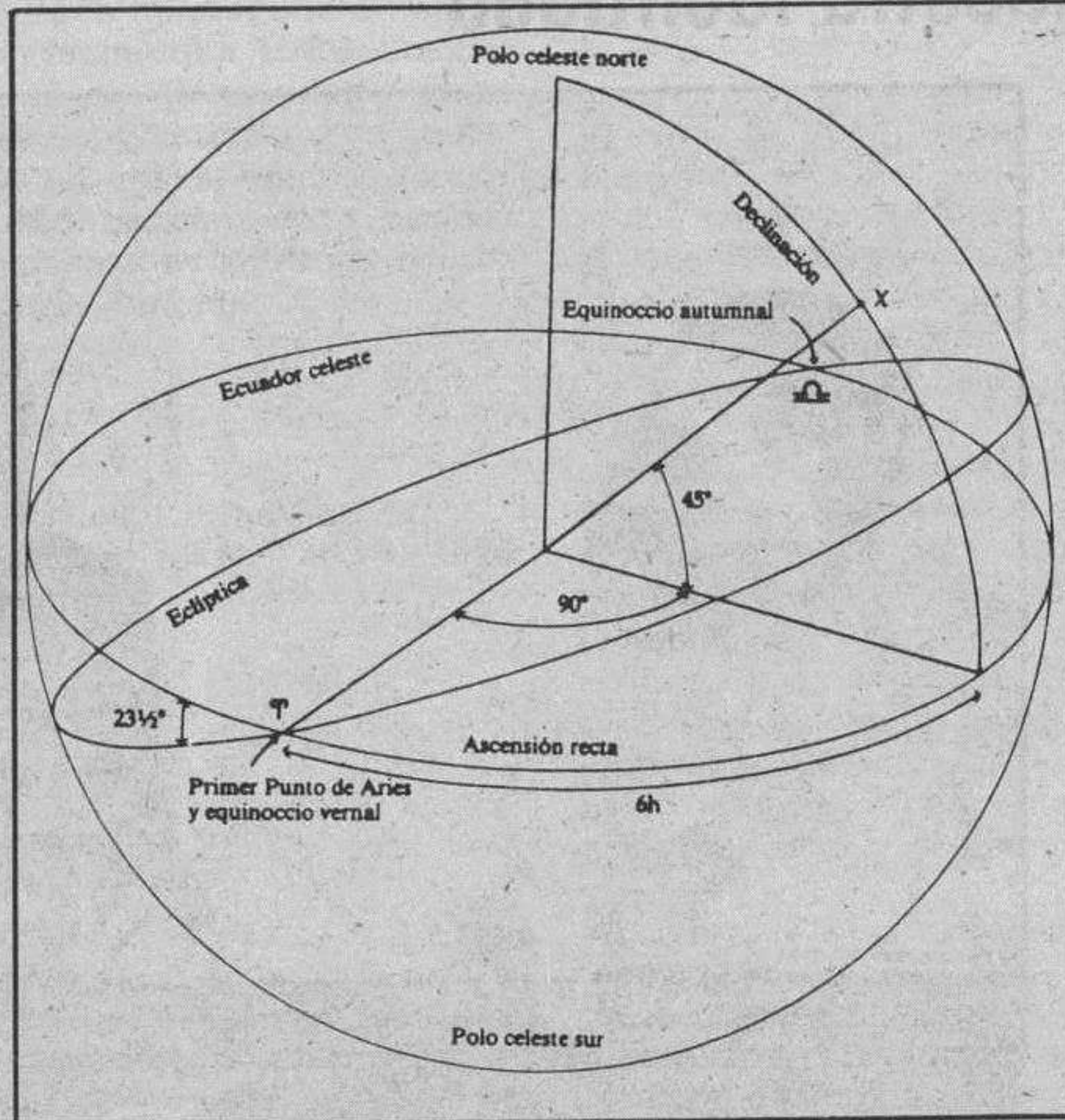
Coordenadas Celestes. El punto X se encuentra a 45° de declinación, y a 6 horas de ascensión recta. La eclíptica es el recorrido aparente del Sol, y tiene 23,5° de inclinación con respecto al Ecuador Celeste debido a la inclinación del eje de la Tierra, que estaría en el centro de esta esfera. La eclíptica corta al Ecuador Celeste en dos ocasiones cada año: los equinoccios (21 de Marzo y 21 de Septiembre).
