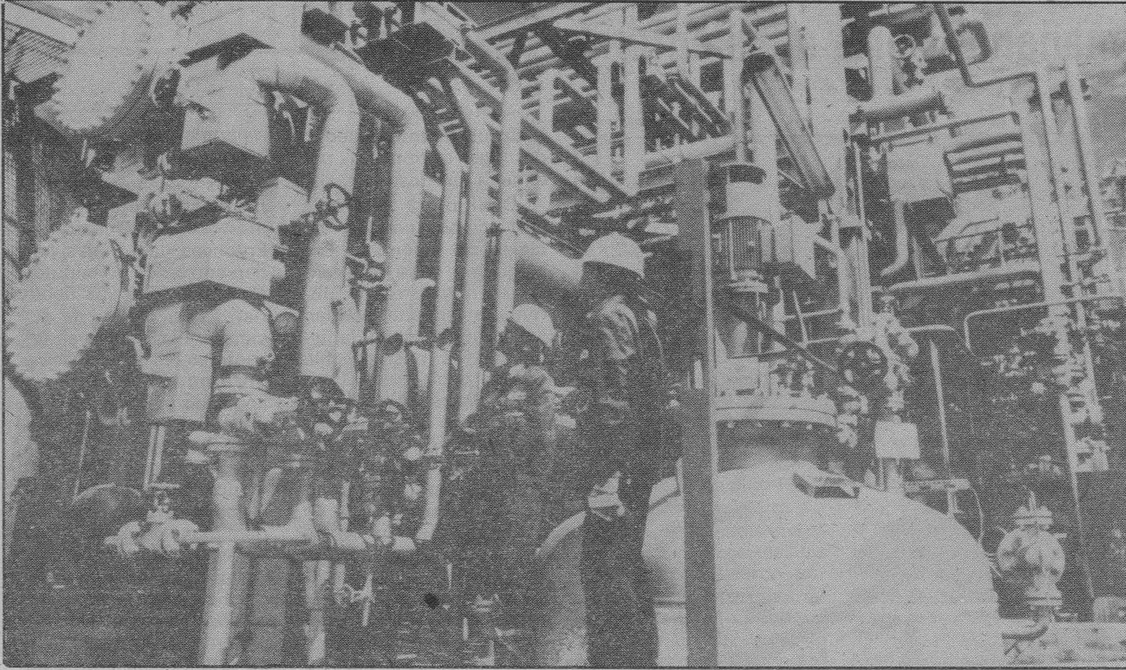
Gasolina sin plomo. — En la fotografía, la planta de eterización o impregnación con eter para la elaboración de gasolina sin plomo construida por el consorcio industrial Krupp Koppers GmbH, de Essen (República Federal de Alemania), en la localidad de Vohburg. La planta eteriza mediante un nuevo método desarrollado por Krupp Koppers el octanaje de los componentes básicos del combustible, gasolina ligera cracking, de butileno y metanol. La eterización en fase líquida, a través de catalizadores, genera un producto de alta calidad que facilita la producción de gasolina sin plomo.
