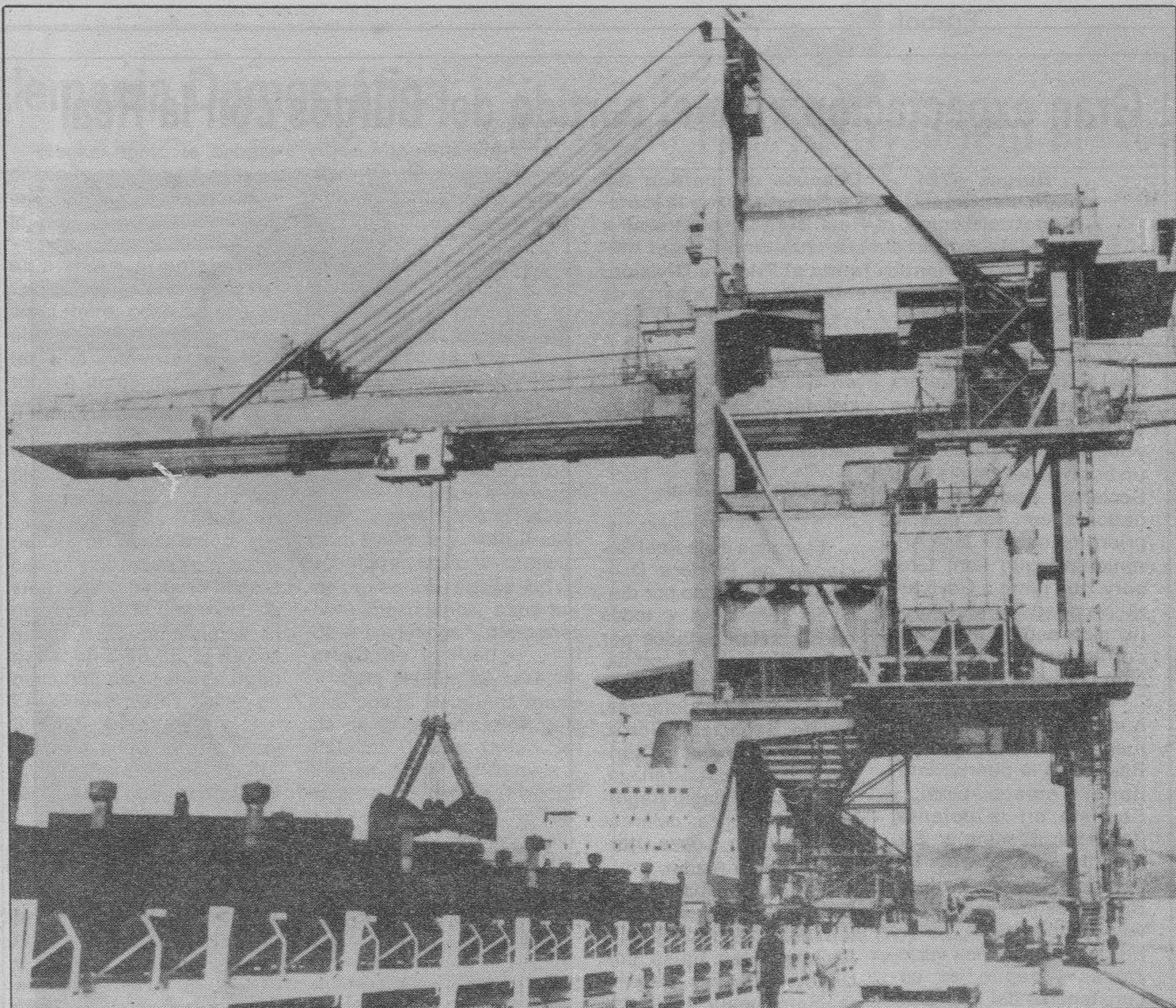
Grúa especial. — En el puerto de Carboneras (España), ha entrado en servicio una moderna instalación para la descarga de barcos carboneros con una capacidad de movimiento de 1.500 toneladas/hora. Ha sido construida esta grúa especial por el consorcio Krupp (República Federal Alemana) y Astilleros y Talleres del Noroeste, S.A., del Ferrol. La particularidad estriba en que la descarga se realiza a través de mando automático. El conductor de la grúa se limita a controlar la operación.
