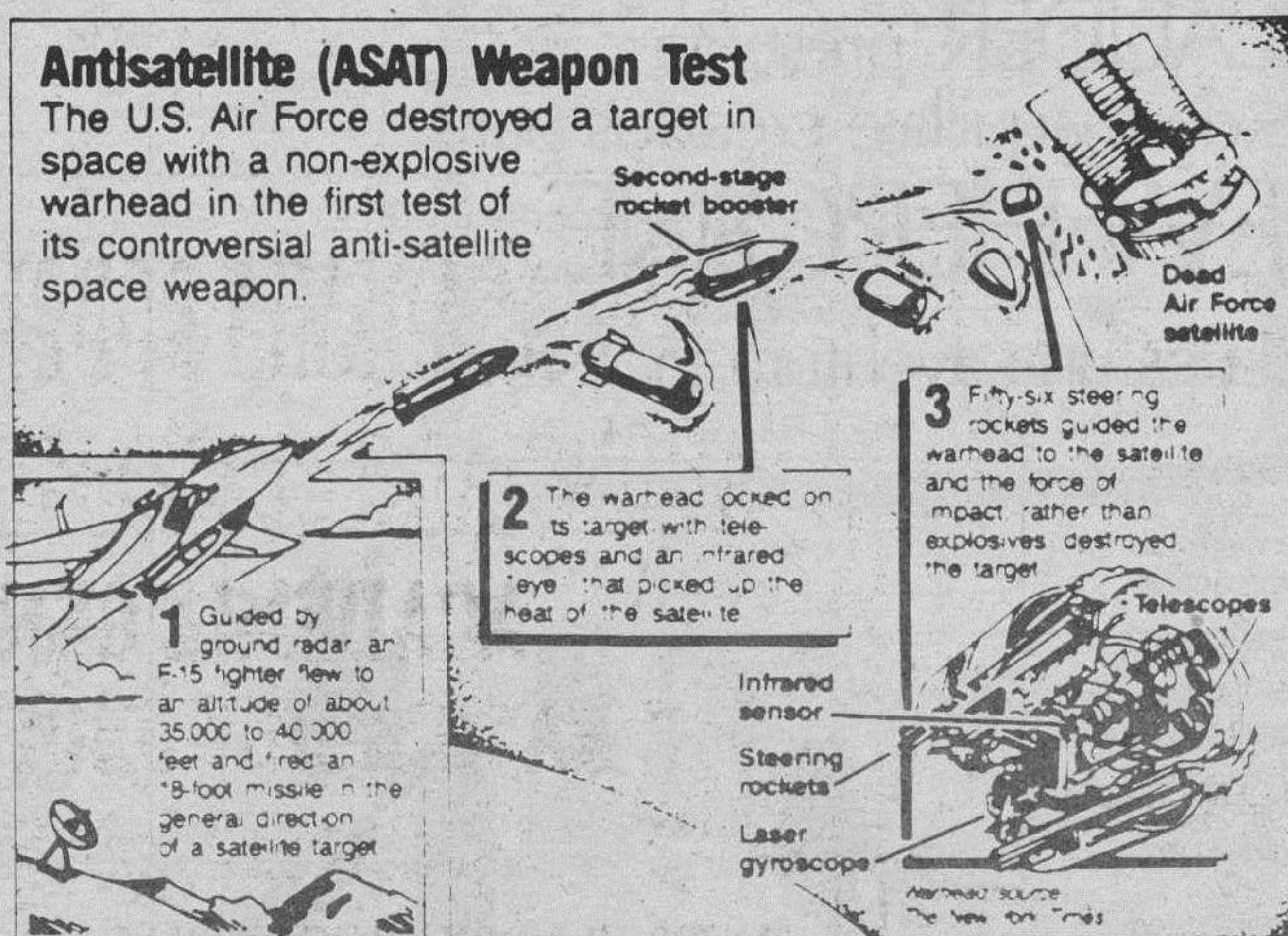
Esquema del funcionamiento del ASAT: el misil es lanzado desde un avión F-15. Dirigido con infrarrojos, en la primera fase se desprende de los cohetes propulsores. En una segunda fase, la cabeza del misil alcanza al satélite y lo destruye.
